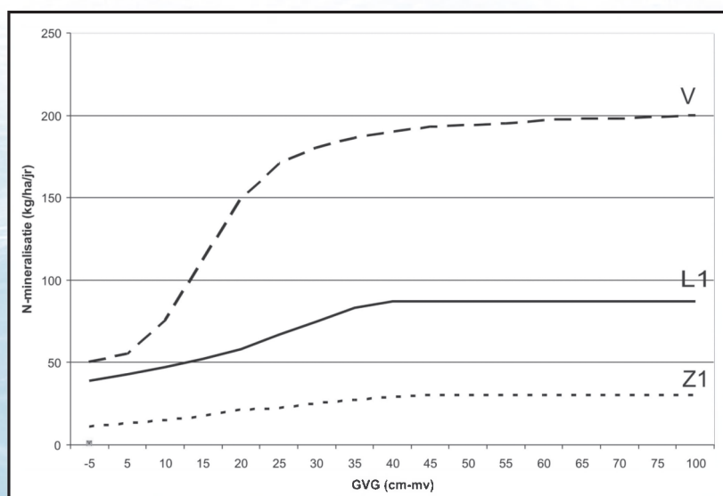
Figuur 3: Mineralisatiecurven van humusarm zand (Z1), alluviale leemgronden met weinig organisch materiaal (L1) en veen (V) in functie van de gemiddelde voorjaarsgrondwaterstand (GVG) uit NICHE Vlaanderen (Callebaut et al. 2007).
