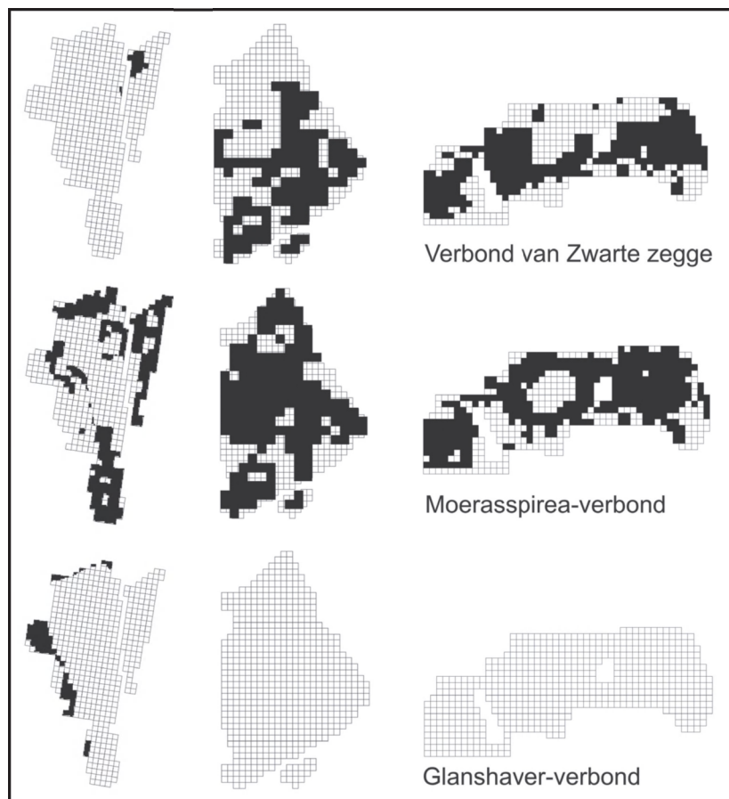
Figuur 7: De berekening van enkele vegetatietypes in drie testgebieden. Van links naar rechts Dooide Bemde, Vorsdonkbos-turfputten en Vallei van de Zwarte Beek.
