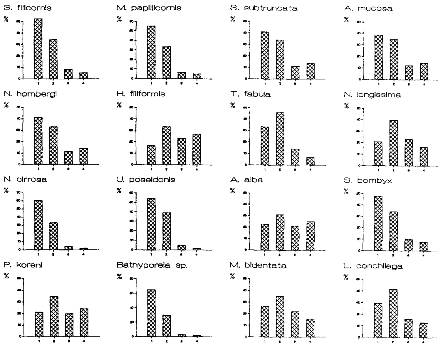
Figuur 28: Habitatspreferentie (slibgehalte) van enkele dominante makrobenthossoorten in de Voordelta.
