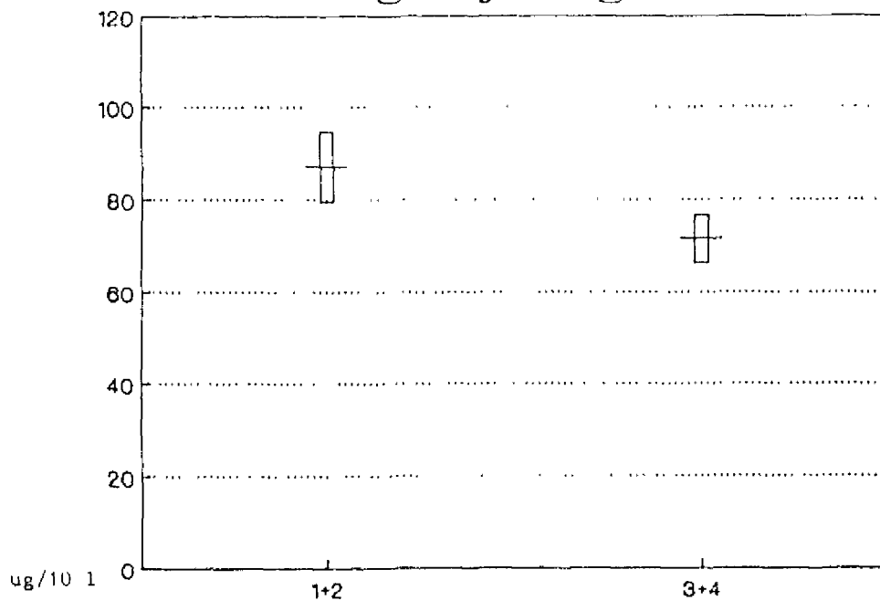
Figuur 6 : Vergelijking van de maximale stroomsnelheid (Vmax) (a) van de zes twinggroepen en het chl a gehalte ( \mu\text{g}/10\text{ l} ) (b) van de twee twinggroepen onderscheiden op basis van de nematodengemeenschappen in de Voordelta (gemiddelde waarde \pm standaardfout).
