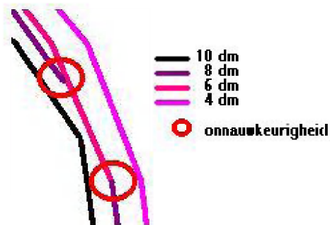
Figuur 7.1: Onnauwkeurigheden in hoogtelijnen
