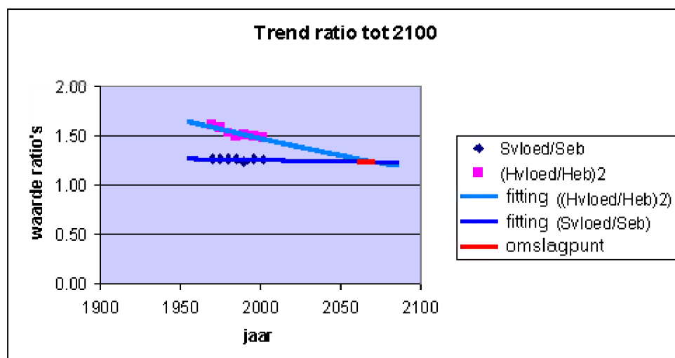
Figuur 1b: trend ratio wateroppervlak en waterdiepte bij vloed en eb. De trends snijden in 2060. Dit impliceert het systeem omslaat van sedimentierend naar eroderend.
