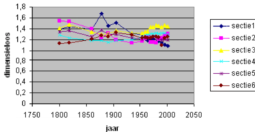
Figuur 6.10: Ratio Wateroppervlak
