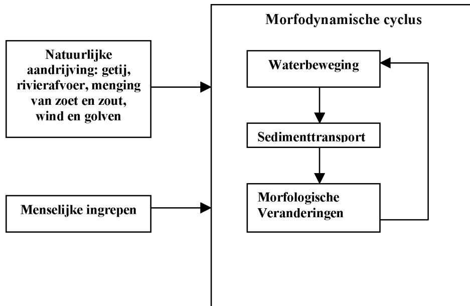
Figuur 5.2 Morfodynamische cyclus (Schippers, 2003)
