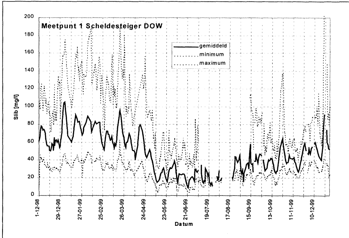
Figuur B1: Verloop van de dubbeldaags-tijgemiddelde slibconcentratie bij meetpunt 1 Scheldesteiger DOW, periode december 1998 - september 1999.
