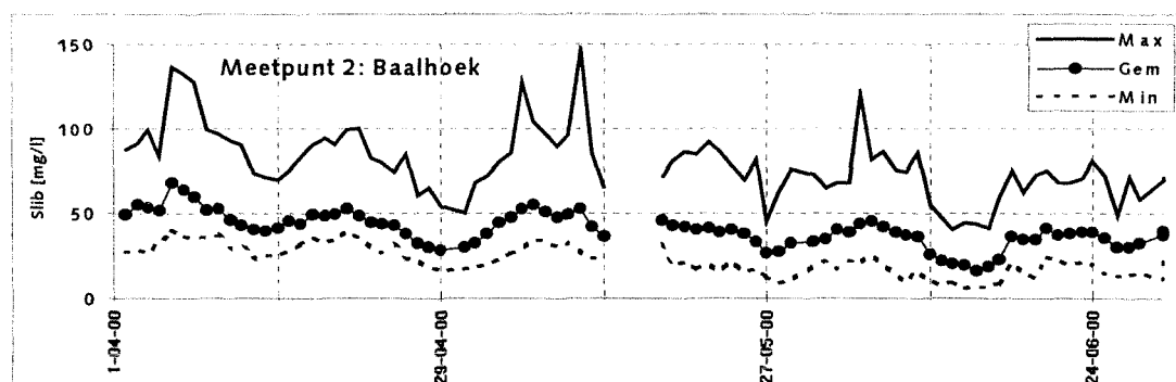
Figuur 6: Verloop van de dubbel-daags-tijgemiddelde slibconcentratie bij Baalhoek, gemiddeld over de waterkolom, periode april - juni 2000. Tevens zijn de minimale en maximale waarden gegeven.
