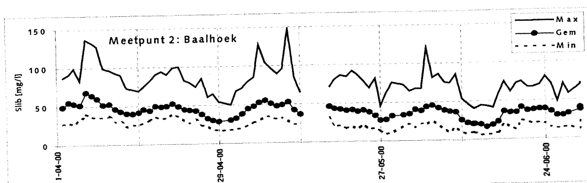
Figuur B4: Verloop van de dubbeldaags-tijgemiddelde slibconcentratie bij meetpunt 2 Baalhoek, periode april - juni 2000.
