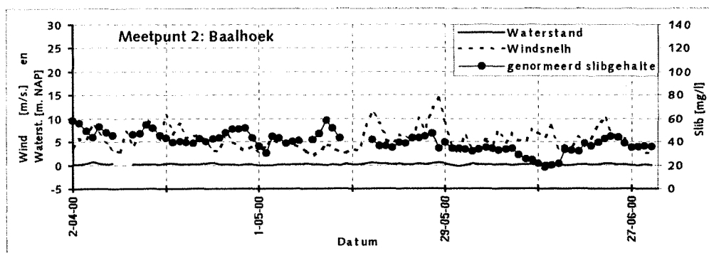
Figuur 8: Genormeed slibconcentratie van meetpunt 2 Baalhoek, waterstand en windsnelheid bij Hansweert periode april - juni 2000.
