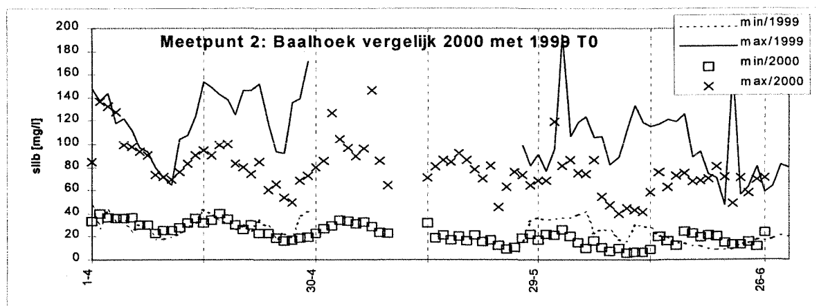
Figuur 12: Vergelijk van de minimale en maximale waarden van de slibconcentratie, behorende bij de dubbeldaags-tijgemiddelde waarden bij Baalhoek, periode april - juni 1999 en 2000.
