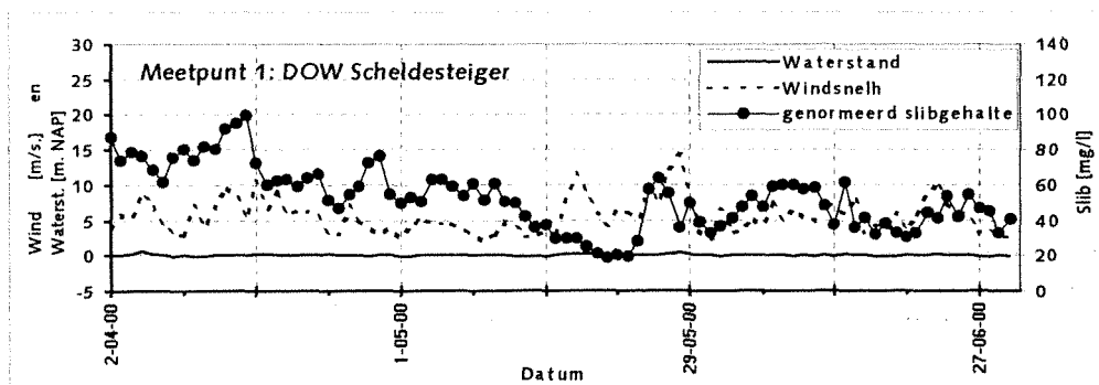
Figuur 7: Genormeed slibconcentratie van meetpunt 1 Scheldesteiger DOW, waterstand bij Terneuzen en windsnelheid bij Hansweert periode april - juni 2000.
