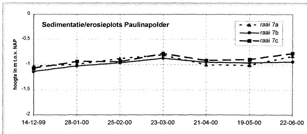
Figuur 13. Gemiddelde veranderingen in de bodemligging van de schorren bij Paulinapolder over de periode januari - juni 2000.
