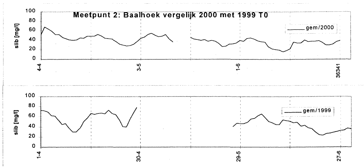
Figuur 11: Vergelijk van de dubbeldaags-tijgemiddelde slibconcentratie bij Baalhoek gemiddeld over de waterkolom, periode april - juni 1999 en 2000.
