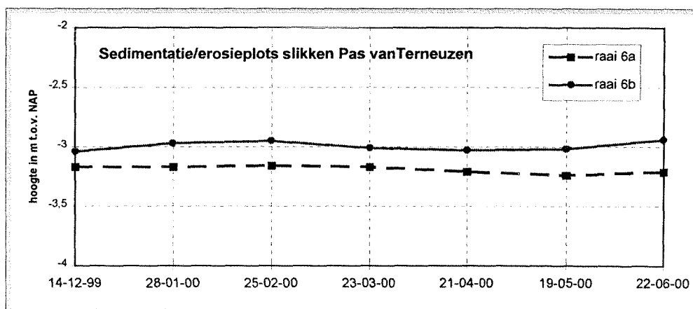
Figuur 14. Gemiddelde veranderingen van de bodemligging van de slikken in het Pas van Terneuzen over de periode januari - juni 2000.
