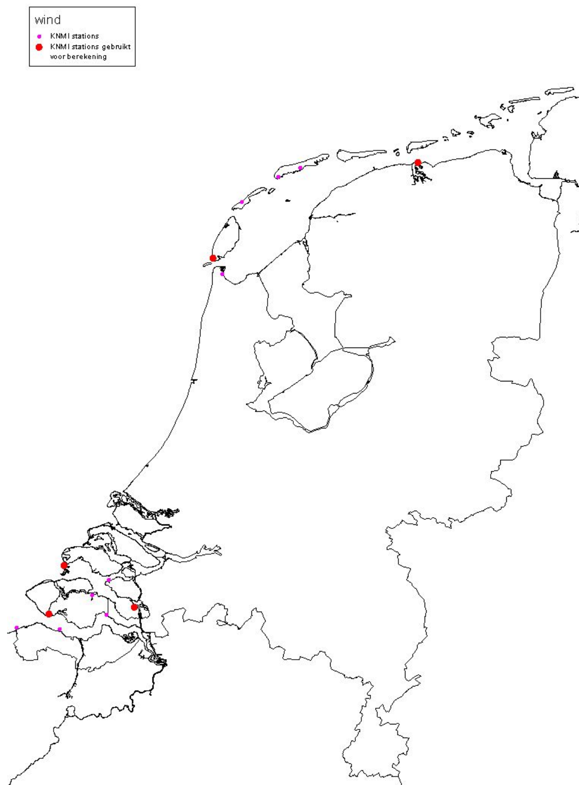
Figuur 2. Locatie stations windgegevens.
