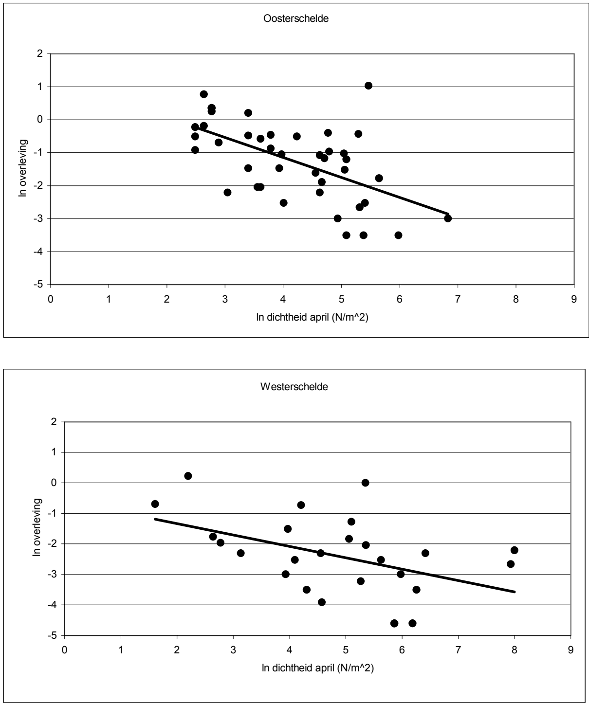
Figuur 1. Relatie tussen de overleving van éénjarige kokkels van april tot april en de dichtheid van éénjarige kokkels in april voor de Oosterschelde en de Westerschelde.
