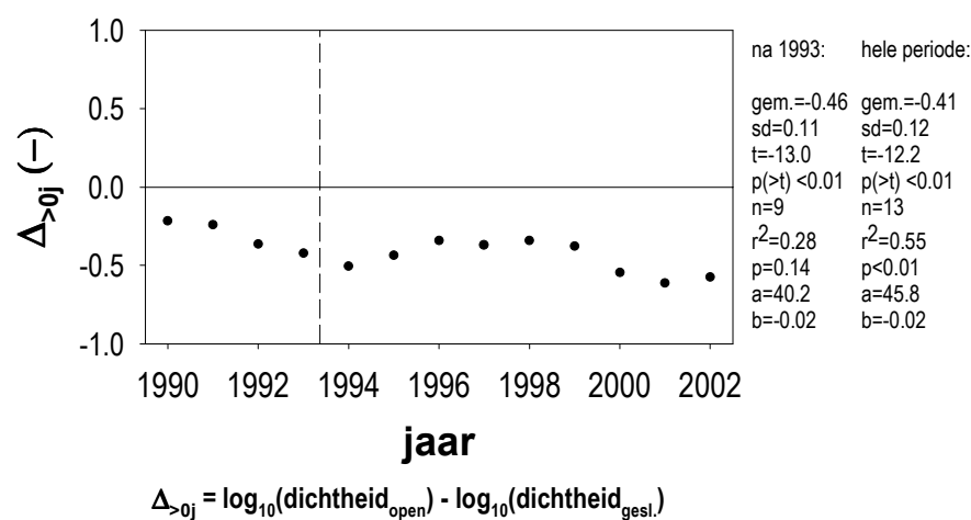
Figuur 4.28. Dichtheden ( \# \cdot \text{m}^{-2} ) kokkels in open versus de in 1993 gesloten gebieden .
