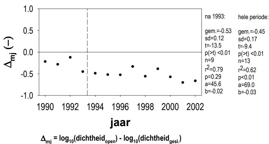
Figuur 4.27. Dichtheden (#.m -2 ) meerjarige kokkels (>1 jaar) in open versus de in 1993 gesloten gebieden .
