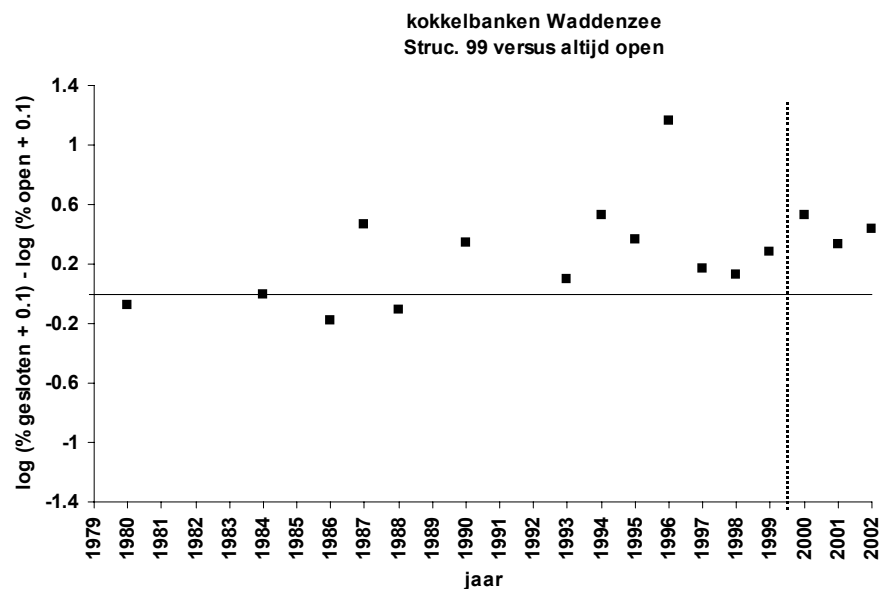
Fig. 2.2. Het verschil in het percentage van het litoraal in de Waddenzee dat is bedekt door kokkelbanken in open en gesloten gebied berekend m.b.v. de gegevens uit tabel 2.2. Een positieve uitkomst geeft aan dat een groter oppervlak aan kokkelbanken in het gesloten gebied aanwezig was en een negatieve uitkomst juist dat er een groter oppervlak aan kokkelbanken in het open gebied aanwezig was. Een aantal jaar is maar deel van de Waddenzee geïnventariseerd en een aantal jaar is in het najaar geïnventariseerd i.p.v. het voorjaar (zie tabel 2.1. voor een overzicht). De locaties van de gebieden zijn weergegeven in figuur 2.1. Hierbij zijn de gebieden uit 1993 die overlap vertoonden met de SBB en Art 17 gebieden alleen meegenomen in de SBB en art. 17 gebieden. Het moment van sluiting is aangegeven met een verticale stippellijn.
