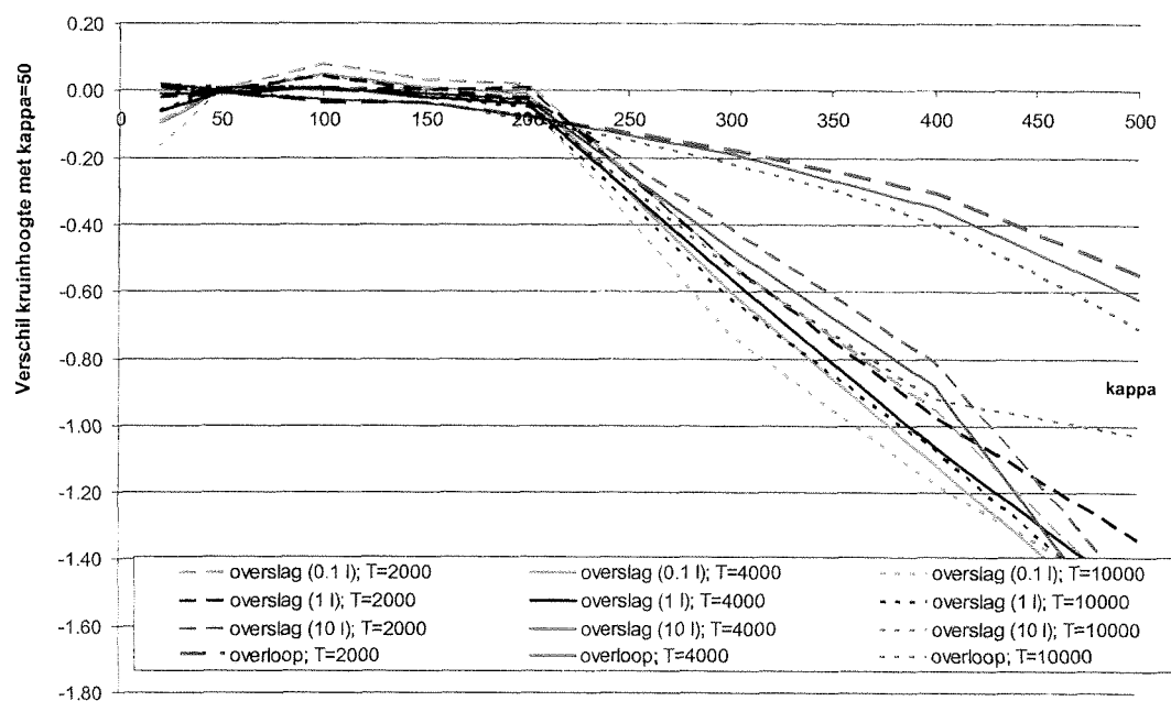
Figuur 7.20 Vershil in dijkhoogte (in [m]) t.o.v. \kappa=50 als functie van \kappa ; locatie Walsoorden
