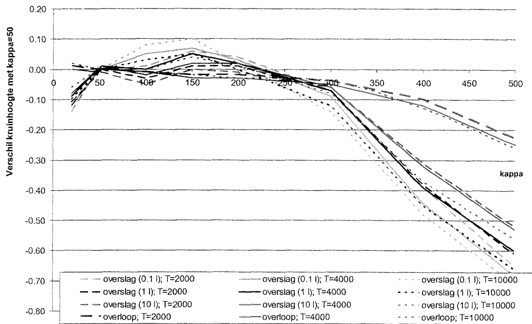
Figuur 7.22 Vershil in dijkhoogte (in [m]) t.o.v. \kappa=50 als functie van \kappa ; locatie Den Helder
