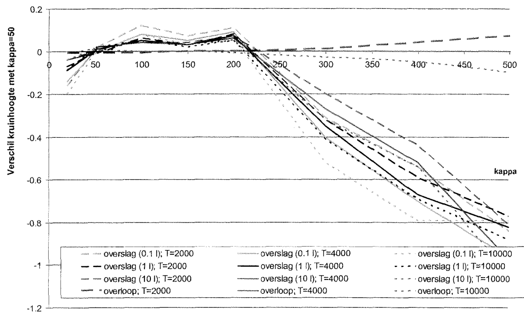
Figuur 7.7 Verschil in dijkhoogte (in [m]) t.o.v. \kappa=50 als functie van \kappa ; locatie Walsoorden
