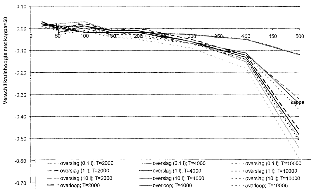
Figuur 7.25 Vershil in dijkhoogte (in [m]) t.o.v. \kappa=50 als functie van \kappa ; locatie Ameland
