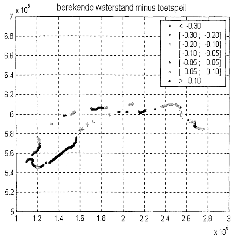
Figuur 2.5 Verschil tussen waterstand en berekend toetspeil voor de Waddenzee
