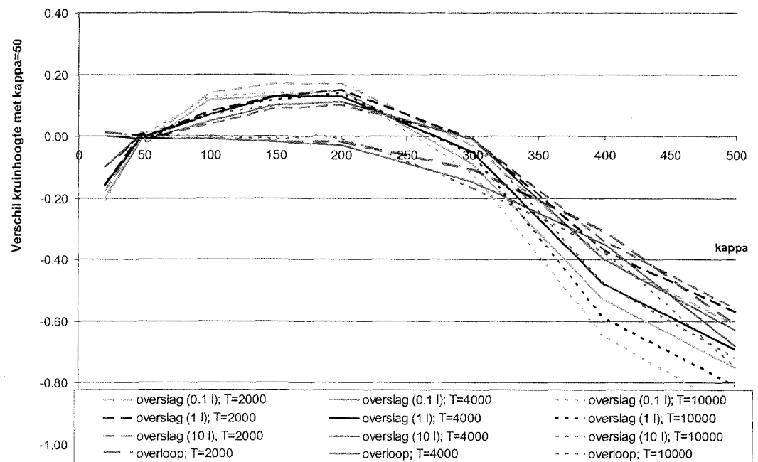
Figuur 7.16 Verschil in dijkhoogte (in [m]) t.o.v. \kappa=50 als functie van \kappa ; locatie Vlissingen
