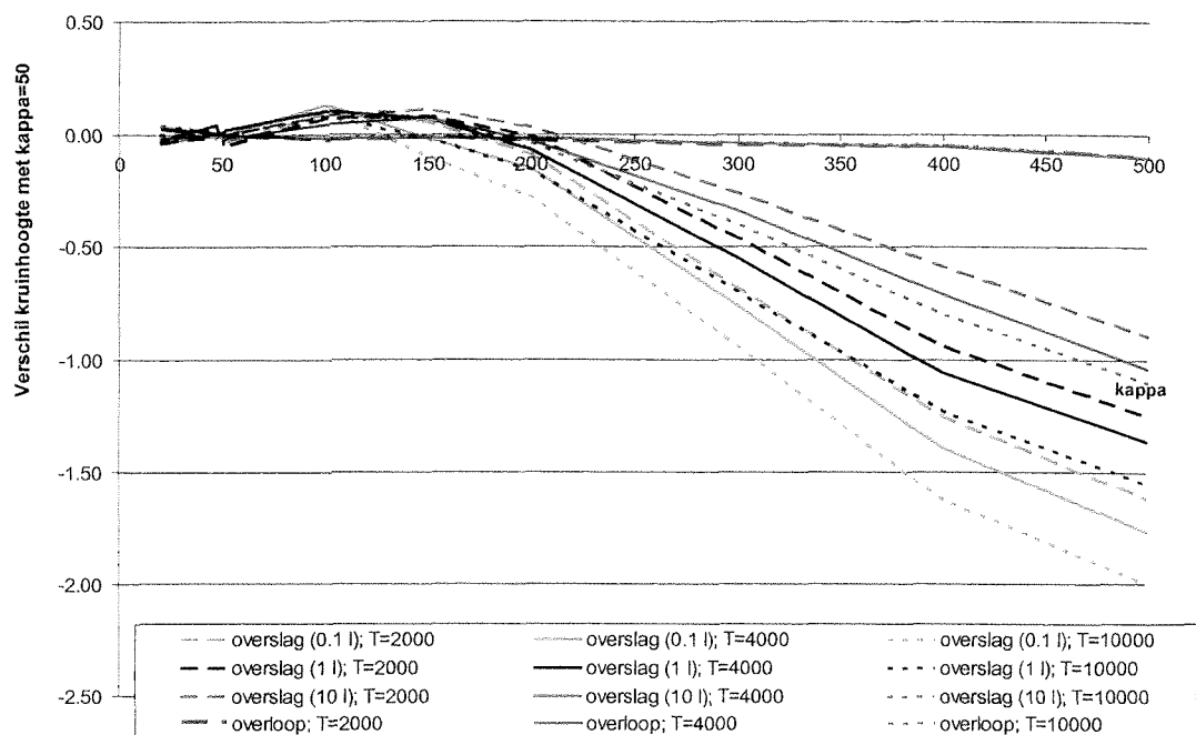
Figuur 7.26 Vershil in dijkhoogte (in [m]) t.o.v. \kappa=50 als functie van \kappa ; locatie Lauwersoog
