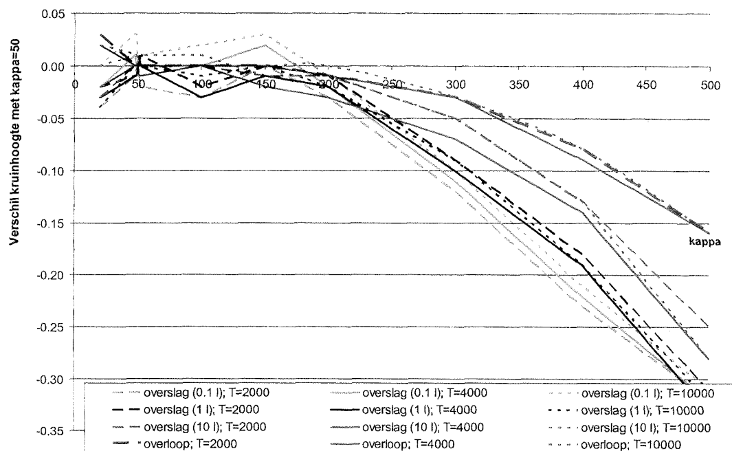
Figuur 7.24 Vershil in dijkhoogte (in [m]) t.o.v. \kappa=50 als functie van \kappa ; locatie Terschelling
