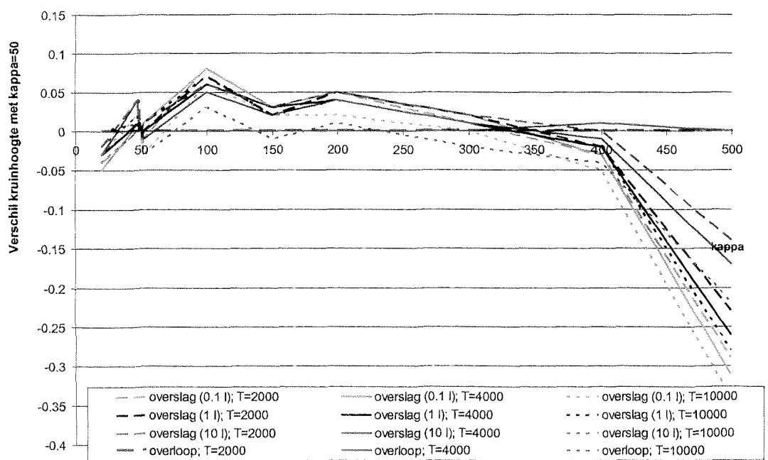
Figuur 7.12 Vershil in dijkhoogte (in [m]) t.o.v. \kappa=50 als functie van \kappa ; locatie Ameland
