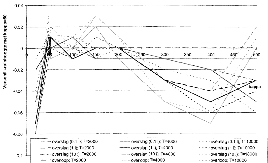
Figuur 7.11 Vershil in dijkhoogte (in [m]) t.o.v. \kappa=50 als functie van \kappa ; locatie Terschelling
