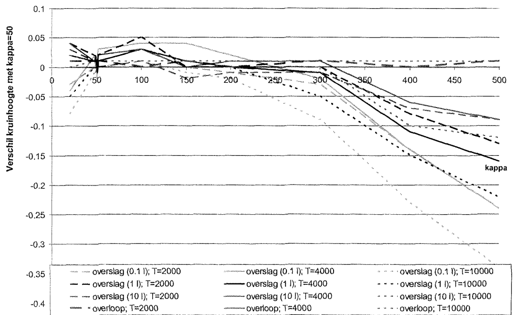
Figuur 7.10 Verschil in dijkhoogte (in [m]) t.o.v. \kappa=50 als functie van \kappa ; locatie Harlingen
