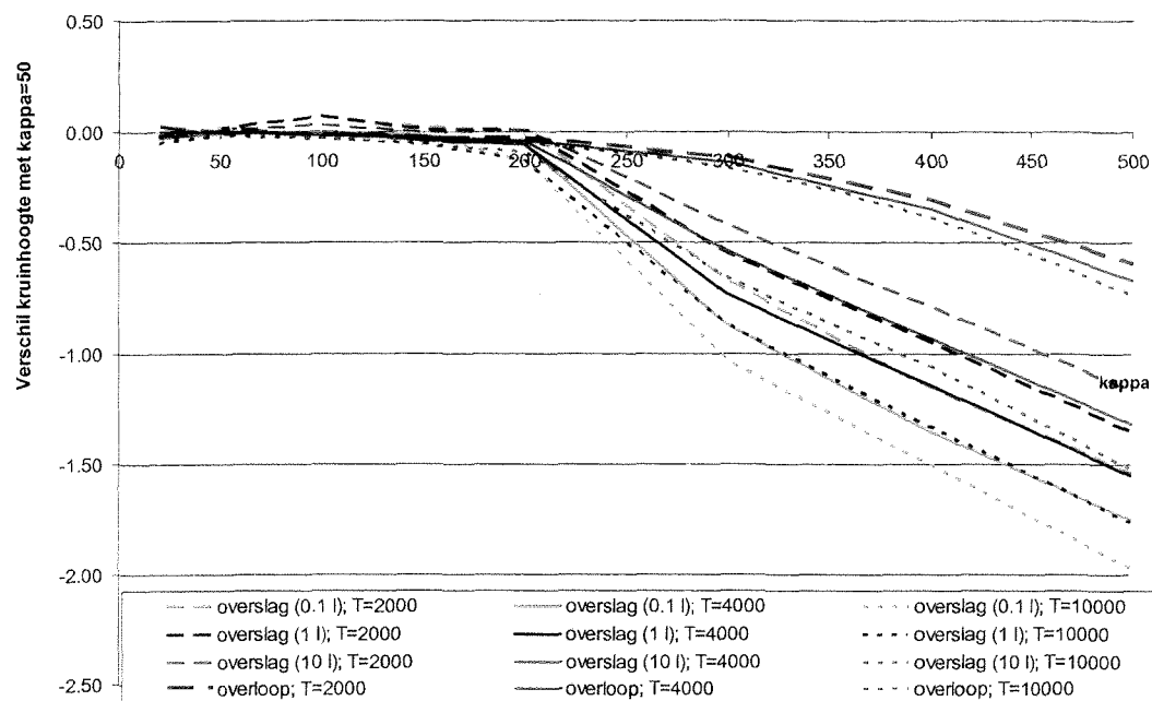
Figuur 7.18 Vershil in dijkhoogte (in [m]) t.o.v. \kappa=50 als functie van \kappa ; locatie Hoofdplaat
