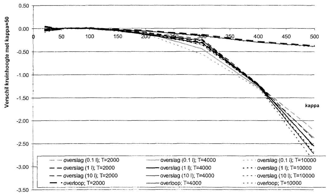
Figuur 7.28 Vershil in dijkhoogte (in [m]) t.o.v. \kappa=50 als functie van \kappa ; locatie Breebaart
