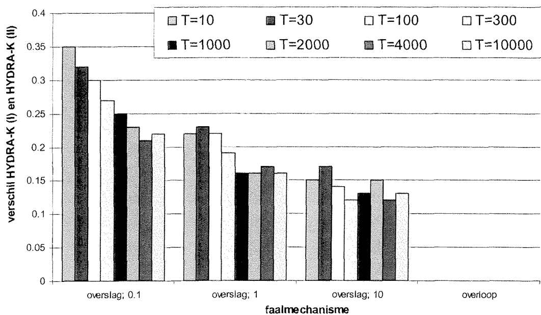
Figuur 7.5 Verschillen in dijkhoogten in [m] door keuze stations (zie Tabel 7.1) voor de locatie Walsoorden.
