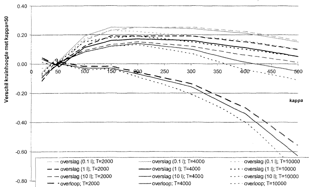
Figuur 7.19 Vershil in dijkhoogte (in [m]) t.o.v. \kappa=50 als functie van \kappa ; locatie Hansweert
