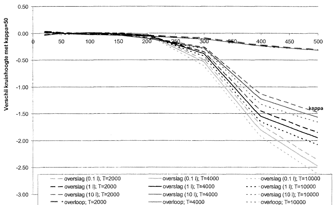
Figuur 7.27 Vershil in dijkhoogte (in [m]) t.o.v. \kappa=50 als functie van \kappa ; locatie Delfzijl
