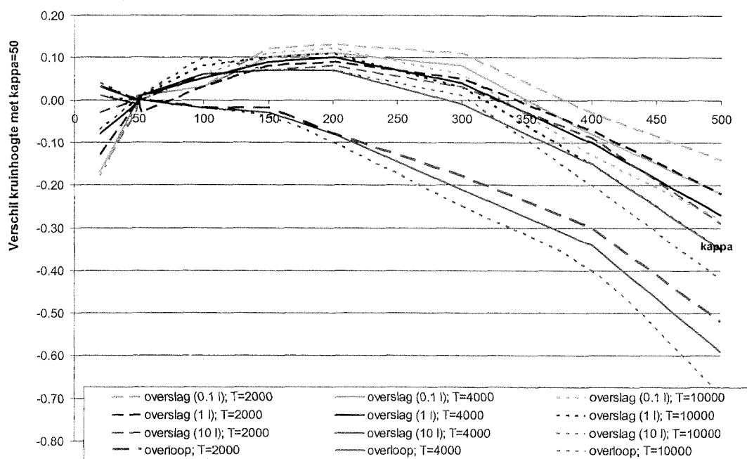
Figuur 7.21 Vershil in dijkhoogte (in [m]) t.o.v. \kappa=50 als functie van \kappa ; locatie Bath
