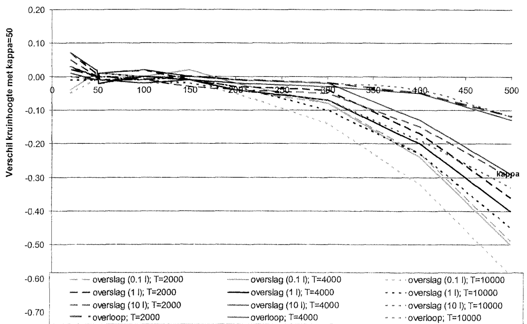
Figuur 7.23 Vershil in dijkhoogte (in [m]) t.o.v. \kappa=50 als functie van \kappa ; locatie Harlingen
