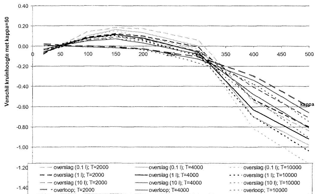
Figuur 7.17 Verschil in dijkhoogte (in [m]) t.o.v. \kappa=50 als functie van \kappa ; locatie Citterspolder
