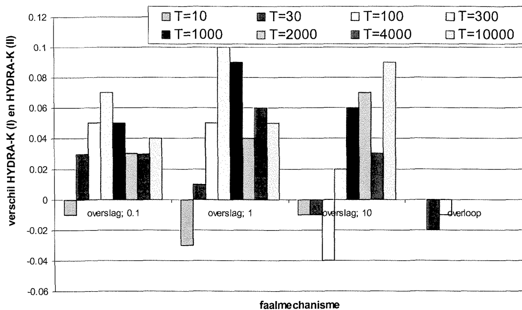
Figuur 7.8 Verschillen in dijkhoogten in [m] door keuze stations (zie Tabel 7.1) voor de locatie Lauwersoog.
