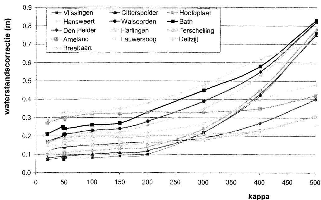
Figuur 7.2 Waterstandscorrecties [m] binnen HYDRA-K als functie van \kappa .
