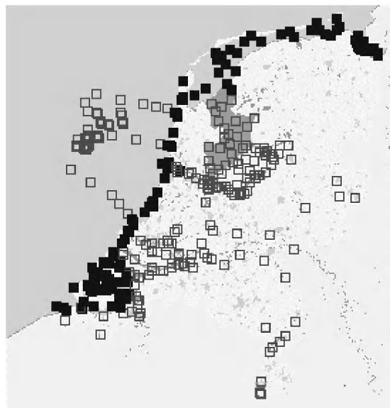
Figuur 2.1 Overzicht van alle meetpunten chlorofyl-a (in \mu\text{g/l} ) in Nederlandse wateren. Meetlokaties met gesloten blokjes zijn geschikt voor de KRW graadmeter voor kust- en overgangswateren.
