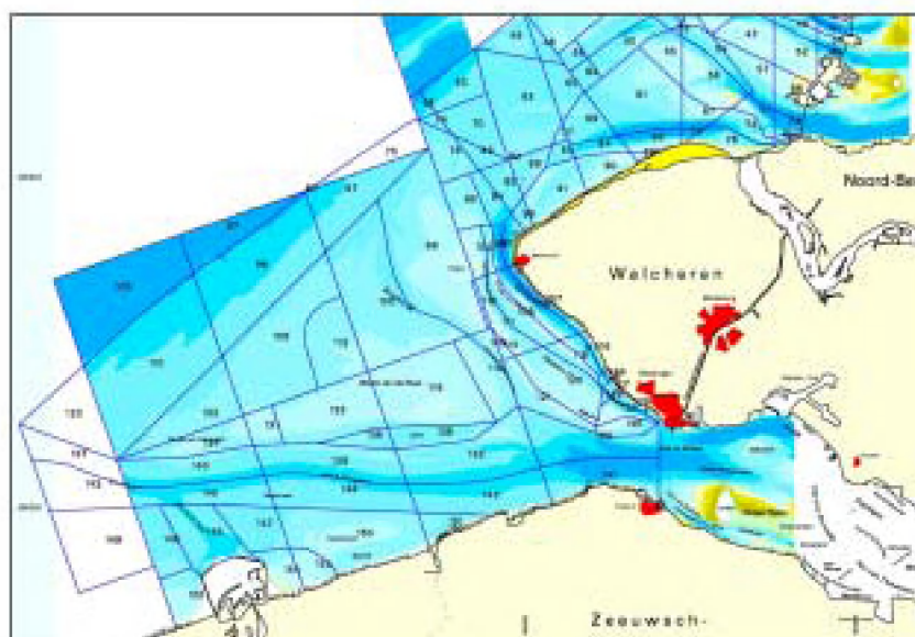
..... Figuur 2.5 Morfologische vakindeling van de monding van de Westerschelde.
