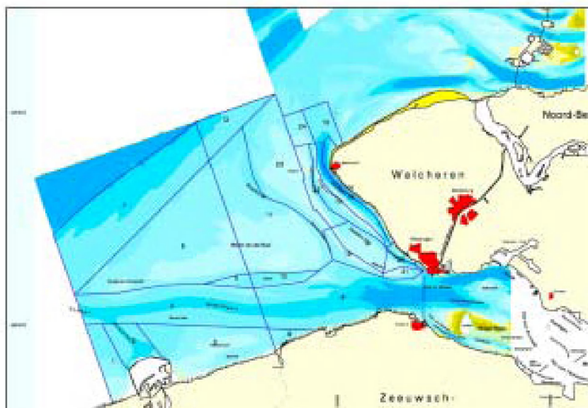
..... Figuur 2.6 Geaggregeerde vakindeling van de monding
