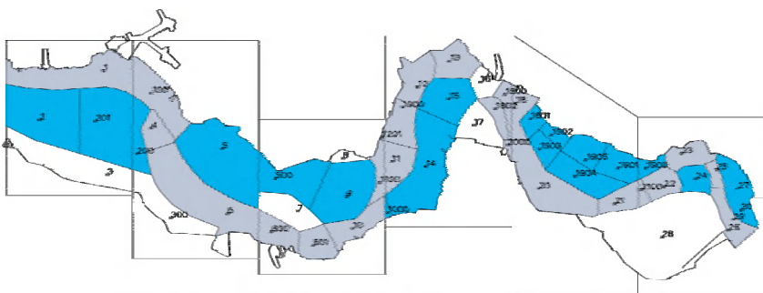
..... Figuur 2.3 Morfologische vakindeling van de Westerschelde. De vloedgeulen zijn donkerblauw weergegeven en de ebgeulen blauwgrijs (zie ook Figuur 2.4). De geulen omvatten ook het grootste deel van de plaatgebieden. De witte vakken maken geen deel uit van een macrocel (zie tekst). De rechthoekige vakken komen overeen met de grenzen van de lodingsvakken.
