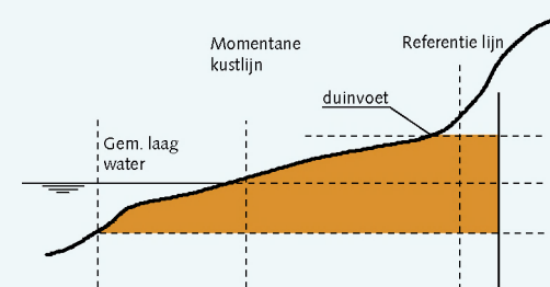
Uit het zandvolume in deze zone wordt jaarlijks de Momentane Kustlijn (MKL) berekend.
