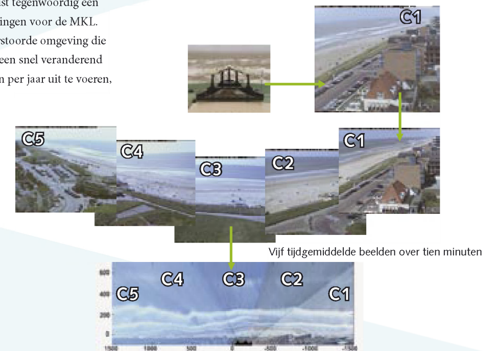
Vijf camerabeelden, via paspunten samengevoegd tot één bovenaanzicht van de kust.
