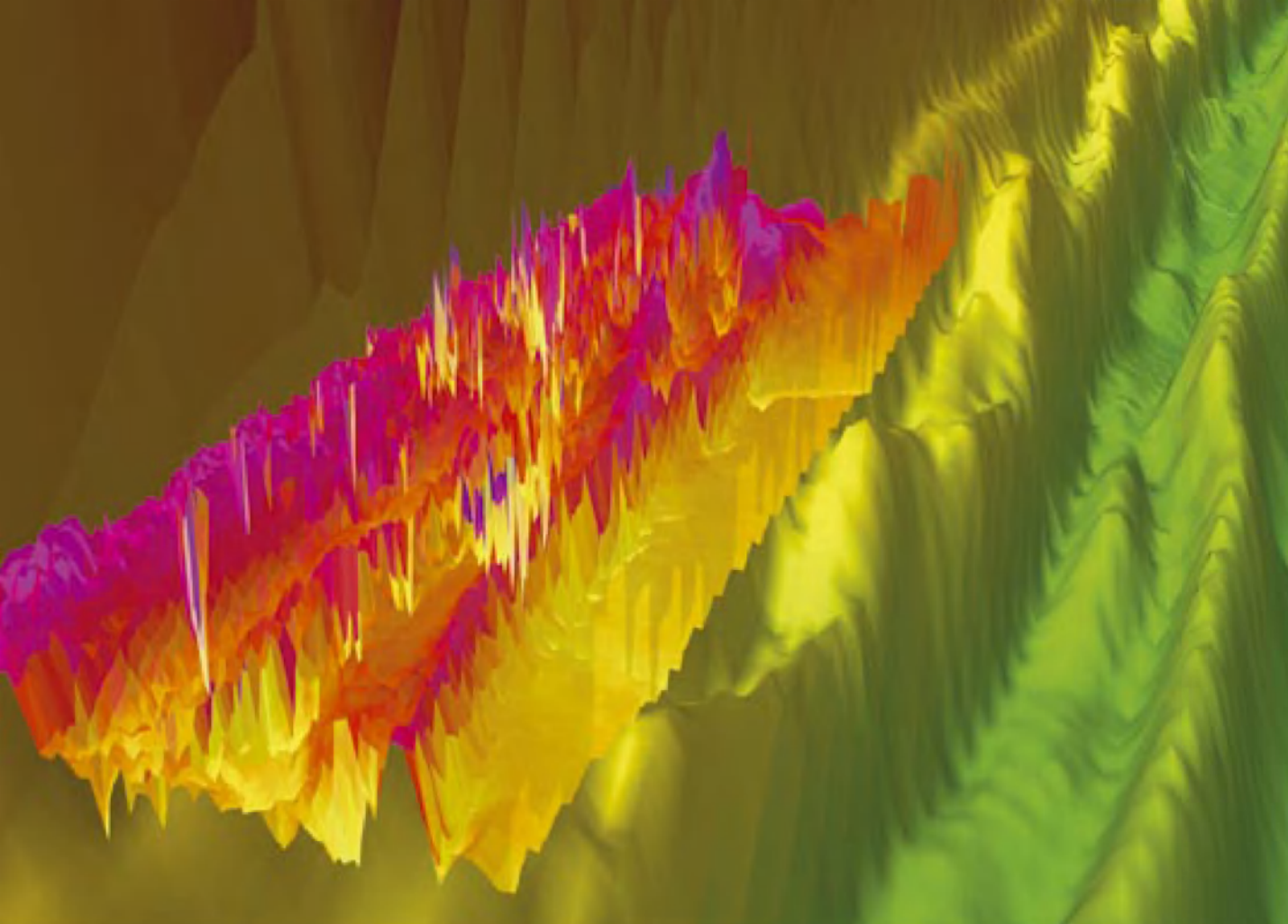
De Argus-videocamera maakt opnames van de plaats waar golven breken. Daaruit is de ligging van de bodem en de kustlijn af te leiden.
