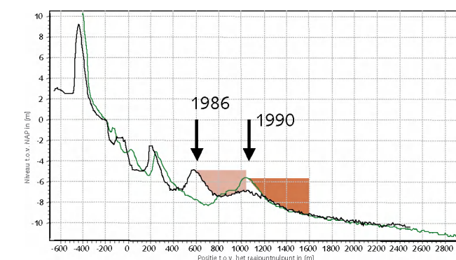
Een onderwatersuppletie (gekleurd) kan op een geschikt tijdstip in de bankencyclus dicht bij de kust worden aangelegd.
