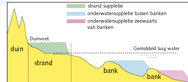
Mogelijke locaties voor suppleties. Tegenwoordig worden onderwater-suppleties meestal zeewaarts van de banken aangelegd.
