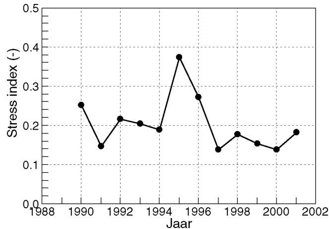
Figuur 3.18. De voedselsituatie van 1998 gecombineerd met het weer en getij van de overige jaren. De strenge winters van 1990–1991, 1995–1996 en 1996–1997 leiden tot extra koudestress.
