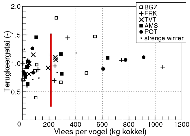
Figuur 3.30. Terugkeergetal voor de deelgebieden (zie Figuur 3.1 op bladzijde 39) als functie van de hoeveelheid niet opgeveste kokkels per vogel. De simulaties voor de deelgebieden zijn onafhankelijk van elkaar. Er is dus geen uitwisseling van vogels of voedsel in het model binnen elk van de winterseizoenen. Voor een voedselvoorraad beneden de 200 kg vlees per vogel bedraagt het gemiddelde terugkeergetal \mu_1 = 0.92 ( n = 23 ). Voor een voedselvoorraad boven de 200 kg vlees per vogel bedraagt het gemiddelde terugkeergetal \mu_2 = 1.07 ( n = 17 ). Het verschil is significant volgens zowel een parametrische t-toets voor de gemiddelden van twee steekproeven met verschillende variantie ( H_0 : \mu_1 = \mu_2 verworpen tegen H_a : \mu_1 < \mu_2 met P=0.040 ) als met de niet-parametrische Mann-Whitney U toets op de medianen ( P=0.035 ).
