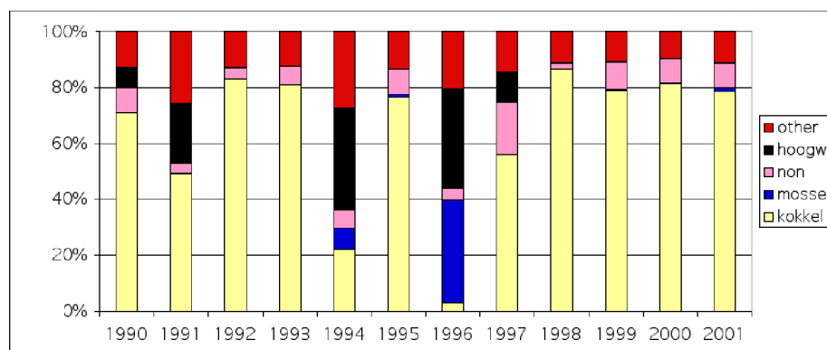
Figuur 5.8. Gesimuleerd diëet voor deelgebied ROT op basis van de historische invoergegevens. Het aandeel nonnetjes is veel kleiner dan gemiddeld voor de hele Waddenzee (zie Figuur 3.7 op bladzijde 49).
