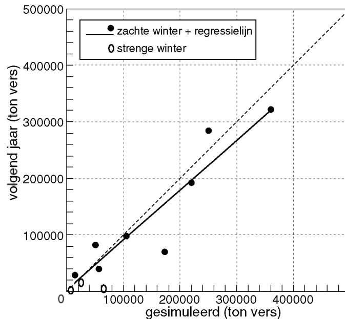
Figuur 3.14. De kokkelbalans voor de Waddenzee met een gesimuleerde hoeveelheid die gecorrigeerd is voor het verschil tussen de bestanden “tussenstand” en “alternatief” in Kamermans et al. (2003b, figuur B1) .
