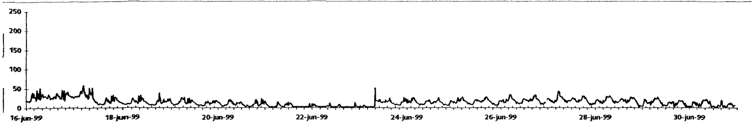
Slibgehalten Terneuzen op NAP - 4,00 m. in mg/l
