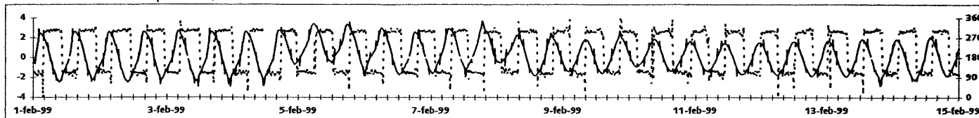
Getij Terneuzen in m. t.o.v. NAP en stroomrichting in graden
