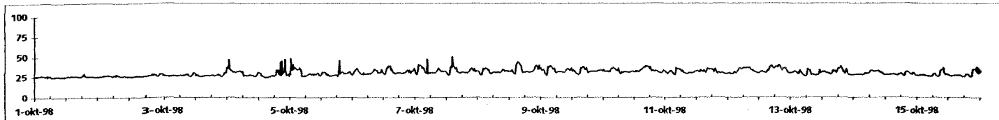
Slibgehalte Vlissingen op NAP-4,50 m. in mg/l
