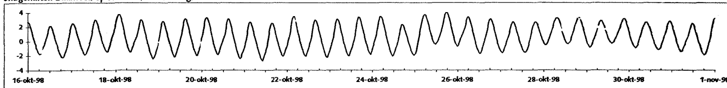
Getij te Baalhoek in m. t.o.v. NAP
