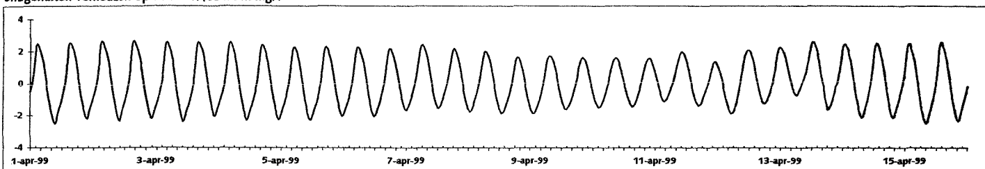
Getij Terneuzen in m. t.o.v. NAP
