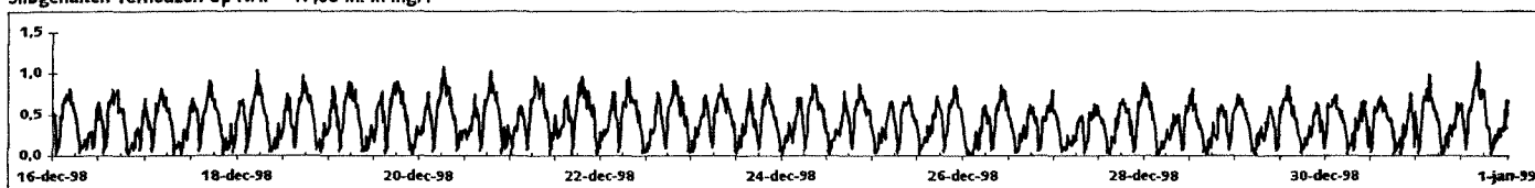
Stroomsnelheid Terneuzen op NAP - 17,00 m. in m./sec.
