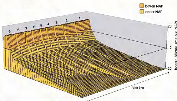
Schematische driedimensionale weergave van onze kust, onderverdeeld in deelsystemen. De cijfers geven de gebiedsaanduiding aan op de kaart van Nederland.
