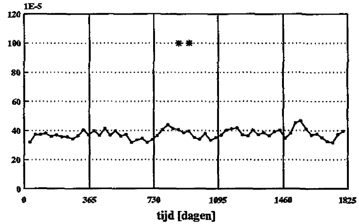
PCB153 totaalconc. waterkolom compartiment 4 [ug/l]
