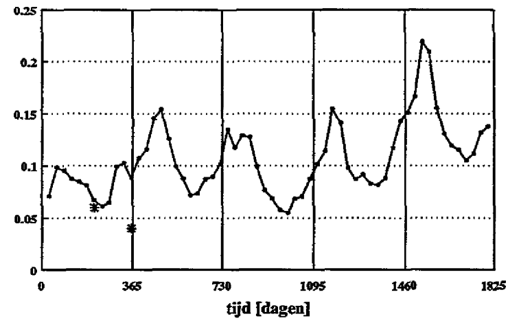
Fla totaalconc. waterkolom compartiment 3 [mg/l]
