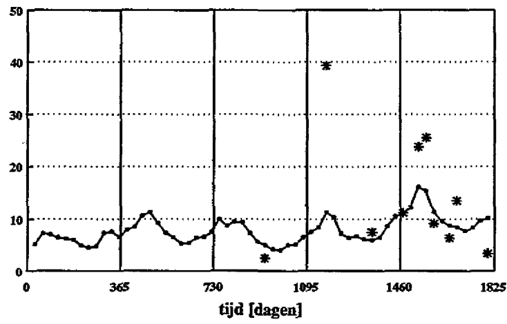
Fla slibkwaliteit waterkolom compartiment 3 [mg/kgOC]
