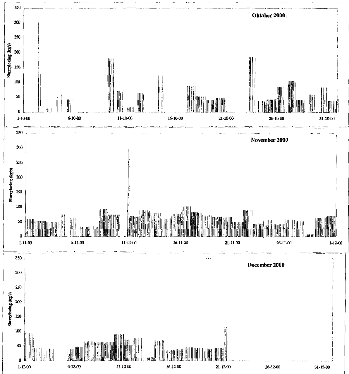
Figuur 3.4 Slurrylozing in de maanden oktober, november en december 2000. Merk op dat de lozing bestaat uit korte pulsen en niet uit langdurige periodes.
