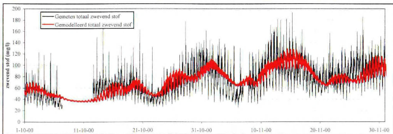
Figuur 4.2 Gemeten en gemodelleerd zwevend stof concentratie op locatie Terneuzen (referentie situatie)
