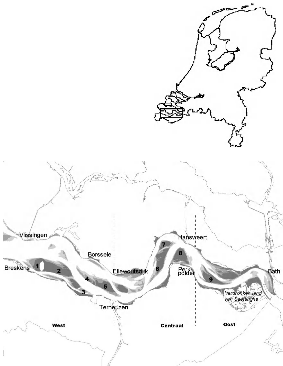
Figuur 1. De Westerschelde met de belangrijkste toponiemen: 1 = Hooge Platen, 2 = Hooge Springer, 3 = Lage Springer, 4 = Suikerplaat, 5 = Middelplaat, 6 = Rug van Baarland, 7 = Brouwerplaat/Molenplaat, 8 = Plaat van Ossenis, 9 = Platen van Valkenisse.
