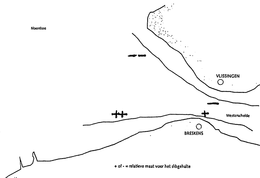
Figuur 9. Kwalitatief beeld van de slibgradiënten in het mondingsgebied van de Westerschelde (naar van Maldegem & Vroon 1995).
