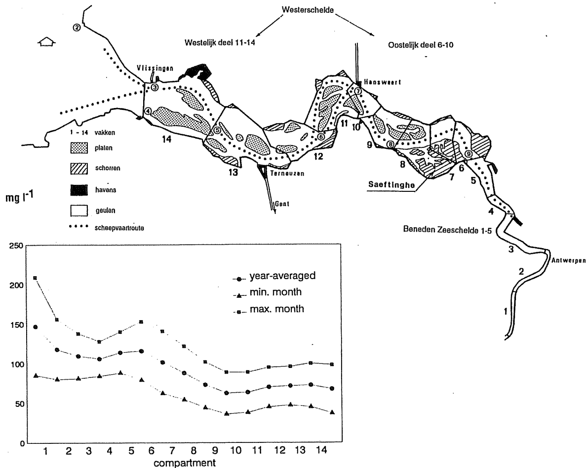
Figuur 8. Diepte- en getijgemiddelde slibconcentratie (fractie < 63 \mu ) op de aangegeven vakgrenzen in de Westerschelde en in de Schelde (van Maldegem et al. 1993)
