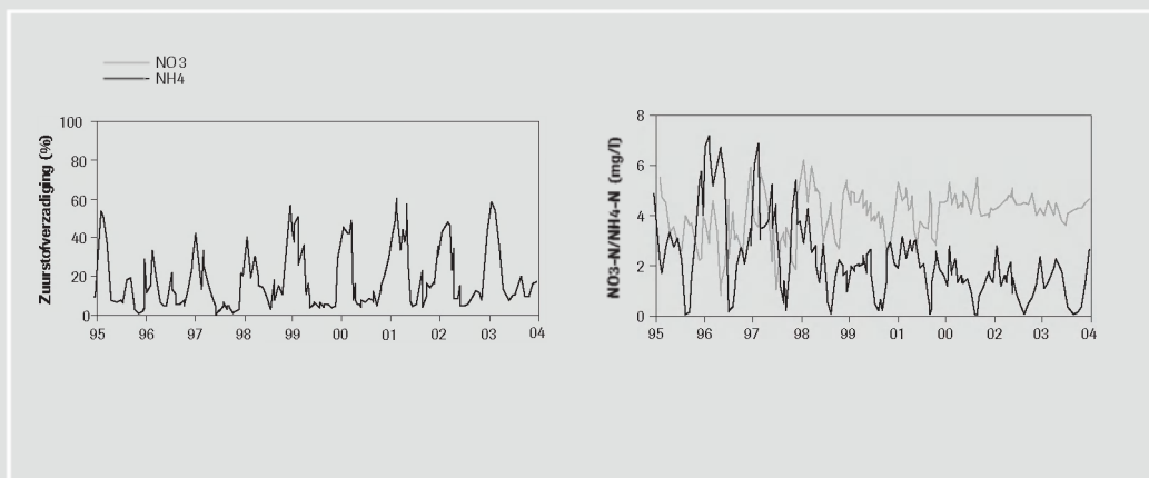
Figuur 14.3: Zuurstofverzadiging (%) en nitraat- en ammoniumconcentraties te Kruibeke over de periode 1995-2003. Op korte termijn waren de zuurstof- en nutriëntenconcentraties beïnvloed door de wisselende neerslag en temperaturen van de voorbije jaren [386].
