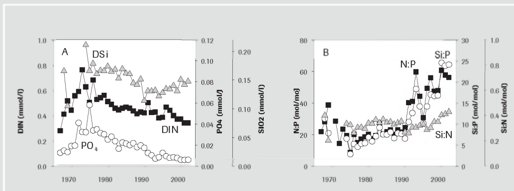
Figuur 14.2: Langtermijnveranderingen in jaargemiddelde eigenschappen van de Zeeschelde ter hoogte van Kruibeke, stroomafwaarts van de Rupelmonding: A. Nutriëntenconcentraties. B. Nutriëntenverhoudingen tussen stikstof (N), fosfor (P) en silicium (Si) (bron: [291]).
