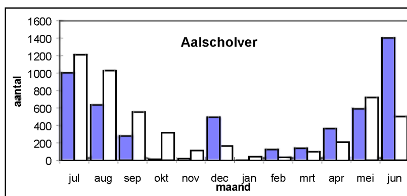
Figuur 6a: Verspreiding van de Aalscholver (gebaseerd op vogeldagen) in de Voordelta in 2000/2001. b: Verdeling over de deelgebieden E=Buitendelta Maasvlakte/Europoort, H=Buitendelta Haringvliet, G=Buitendelta Grevelingenmeer, O=Buitendelta Oosterschelde, W=Westerscheldemonding.
