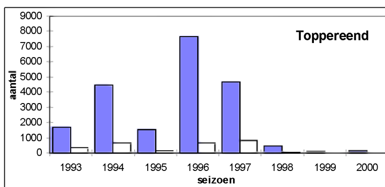
Figuur 11. Seizoensmaxima (gesloten balken) en seizoensgemiddeldes (open balken) van de Toppereend in de Voordelta in de periode 1993/94-2000/2001.
