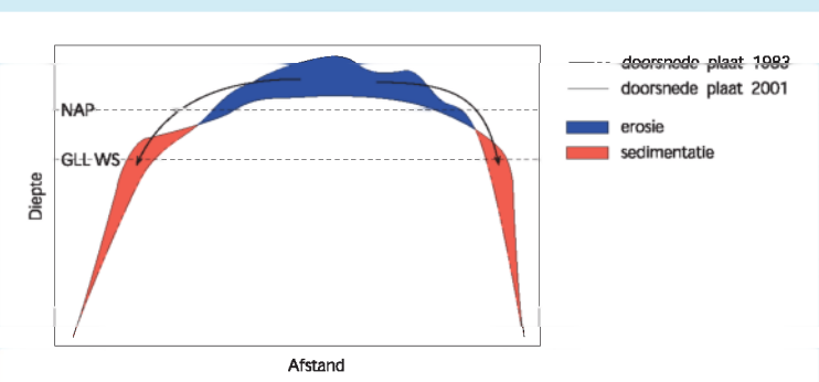
Figuur 2.7 Schematische weergave van het effect van het erosieproces op de ontwikkeling van een plaat in de Oosterschelde.
