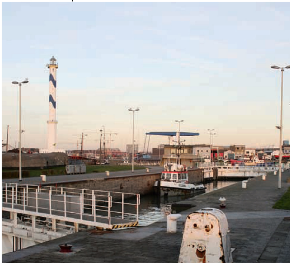
■ De Visserijsluis, die het Visserijdok te Oostende verbindt met de havengeul, is uitgerust met twee paar puntdeuren. Door deze sluis is de achterliggende vissershaven getijvrij (VL)
