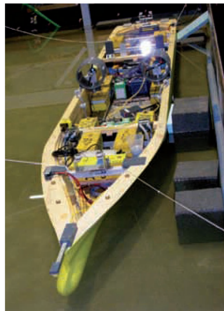
■ Ontwerp van nieuwe sluizen voor het Panama kanaal: Schaalmodelstudie (schaal 1:80) in het Waterbouwkundig Laboratorium te Borgerhout in opdracht van de Autoridad del Canal de Panamá. Zicht op het ontwerpschip (met een capaciteit van 12.000 twintig-voet-containers) met instrumentatie (WL)
