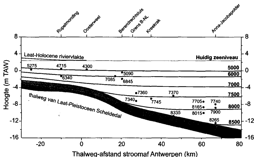
Figuur 8. Evolutie van de riviergradiënt van de Beneden-Schelde in België en Zuidwest-Nederland tijdens het Holoceen. De ouderdommen bij de datapunten geven gecalibreerde ^{14}\text{C} -jaren weer. Voor uitleg zie tekst.
