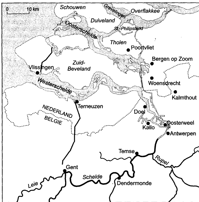
Figuur 1. Het Beneden-Scheldebekken in België en Nederland, met een aantal lokaties vermeld in de tekst. Meer plaatsnamen zijn te vinden op Fig. 3.
