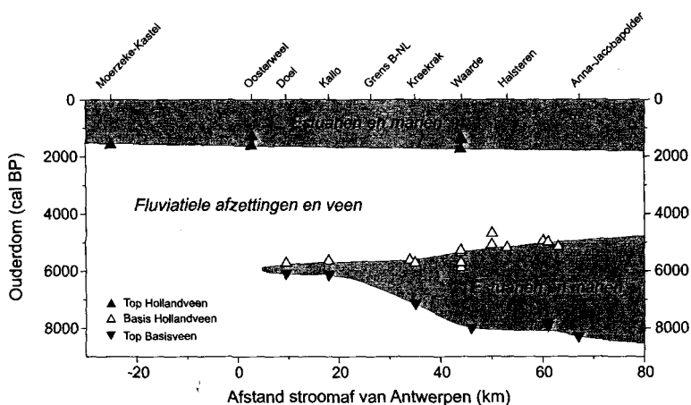
Figuur 6. De Holocene evolutie van de mariene invloed in de Beneden-Schelde in België en Zuidwest-Nederland. Het diagram is gebaseerd op ^{14}\text{C} -dateringen van de boven- en onderkant van regionaal voorkomende veenlagen en fluviatiele en mariene klastische afzettingen, uitgezet in een lengteprofiel langs de rivier. Veen en fluviatiele afzettingen worden gevormd in een terrestrisch en/of zoetwater-afzettingsmilieu, terwijl estuariene en mariene afzettingen een getijden en/of brakwatermilieu voorstellen. De ouderdom is in kalenderjaren voor heden.
