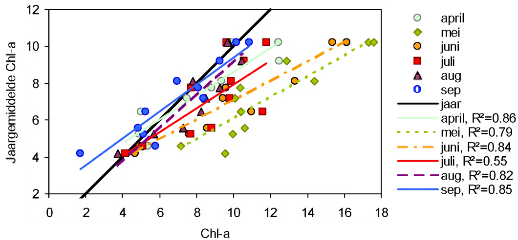
Figuur 26. Relatie tussen maandgemiddelde chlorofyl-gehalte en jaargemiddelde chlorofyl-gehalte (in \mu\text{g/g} ), voor de periode 1993-2003.
