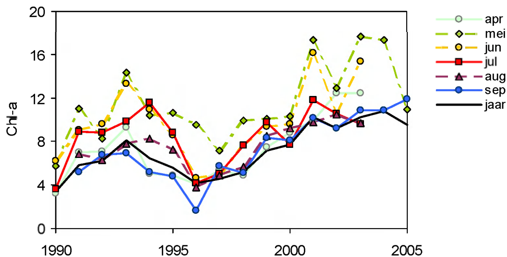
Figuur 27. Temporele variatie van chlorofyl-a aan het oppervlak, uit veldwaarnemingen.
