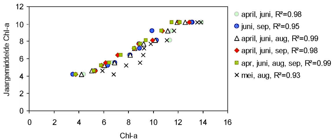
Figuur 29. Relatie tussen meermaandsgemiddelde chlorofyl-gehalte en jaargemiddelde, voor de periode 1993-2003, voor een aantal combinaties.
