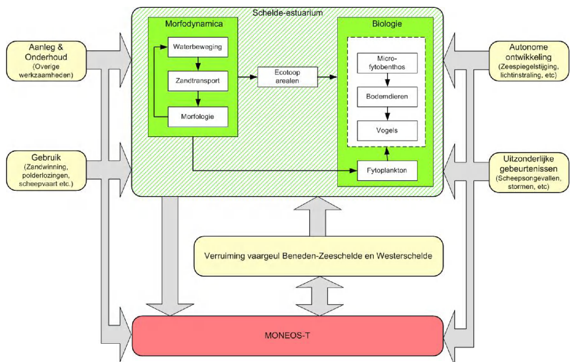
Figuur 5 Systeembeschrijving
