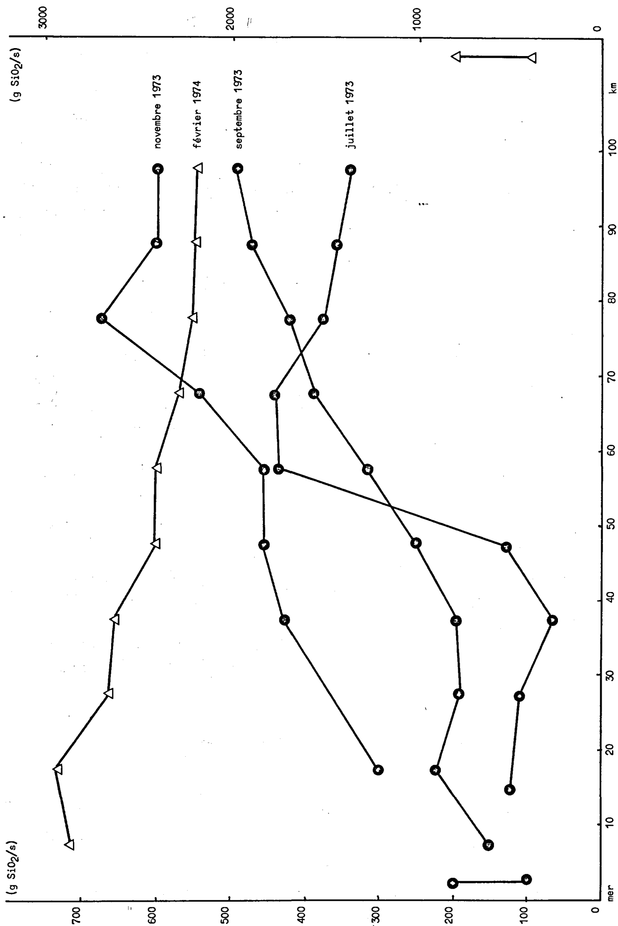
fig. 4. Flux de silice dissoute dans l'Escaut
