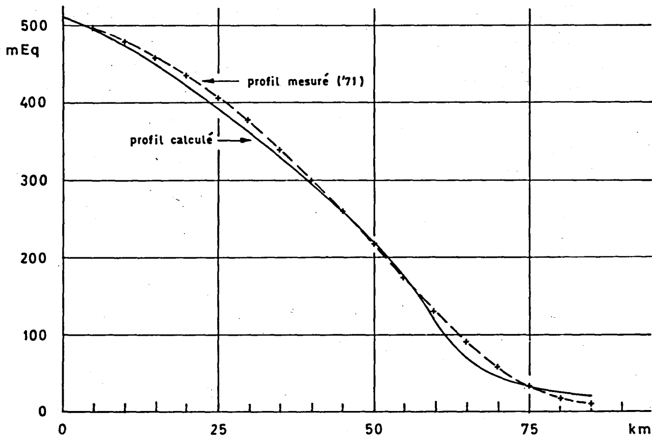
fig. 1a. Calcul des coefficients de dispersion K_x
