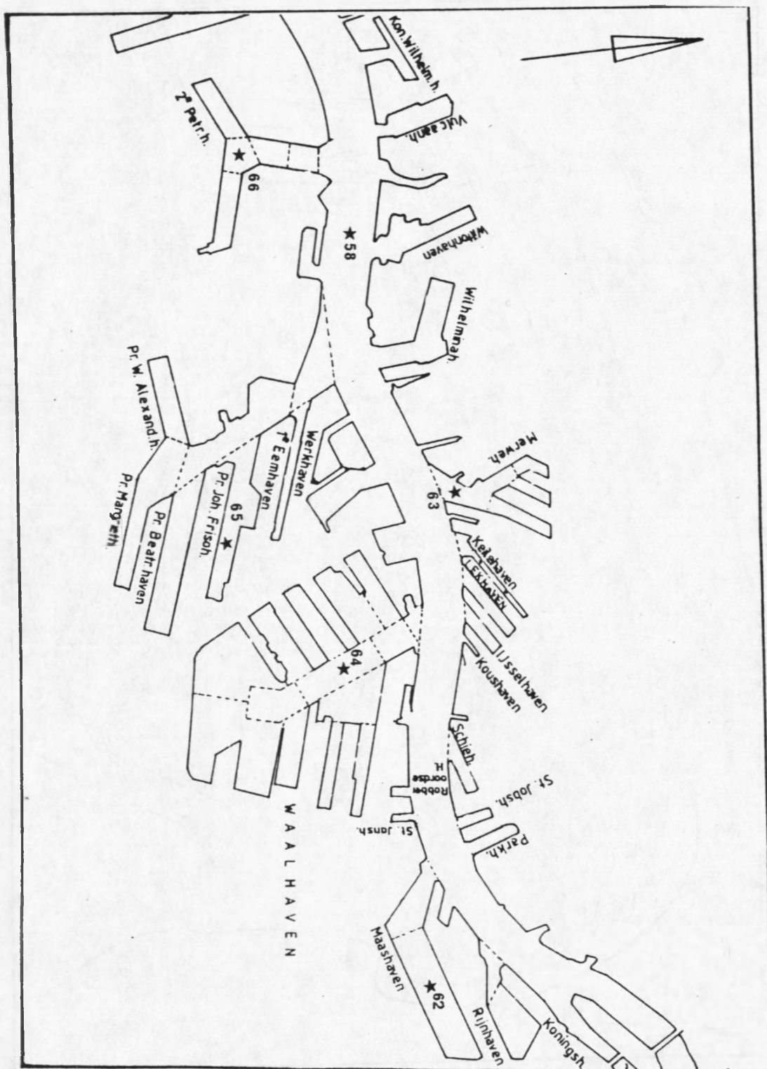
Fig. 7. Sedimentmonster lokaties juni 1986.
