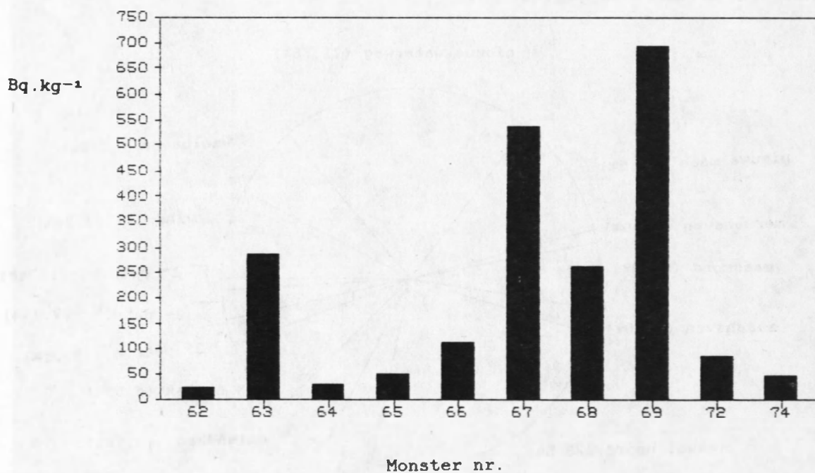
Fig. 21. De ^{210}\text{Po} excess concentraties ( \text{Bq.kg}^{-1} ) in het sediment van het Nieuwe Waterweg gebied.
