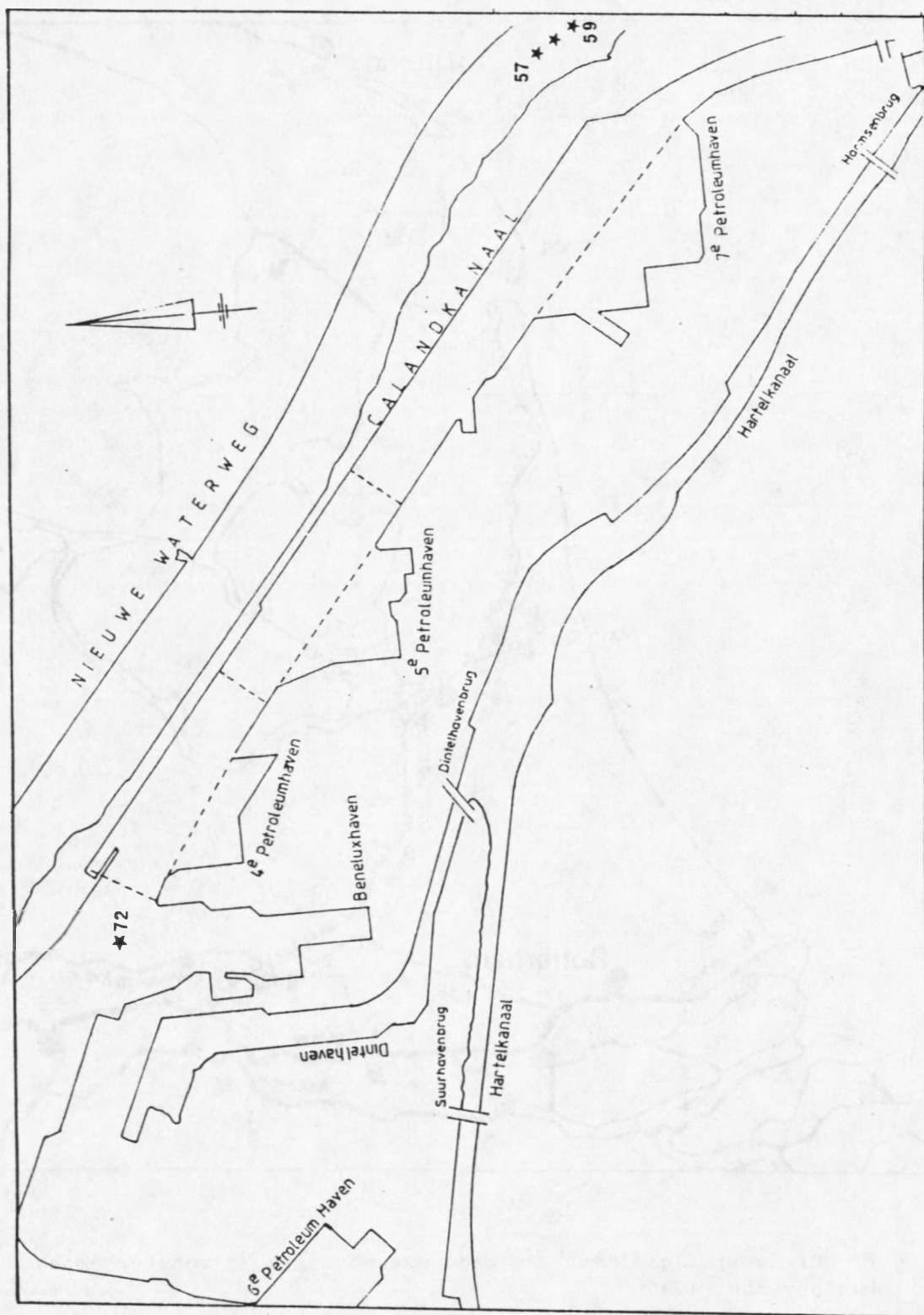
Fig. 3. Sedimentmonster lokaties juni 1986.
