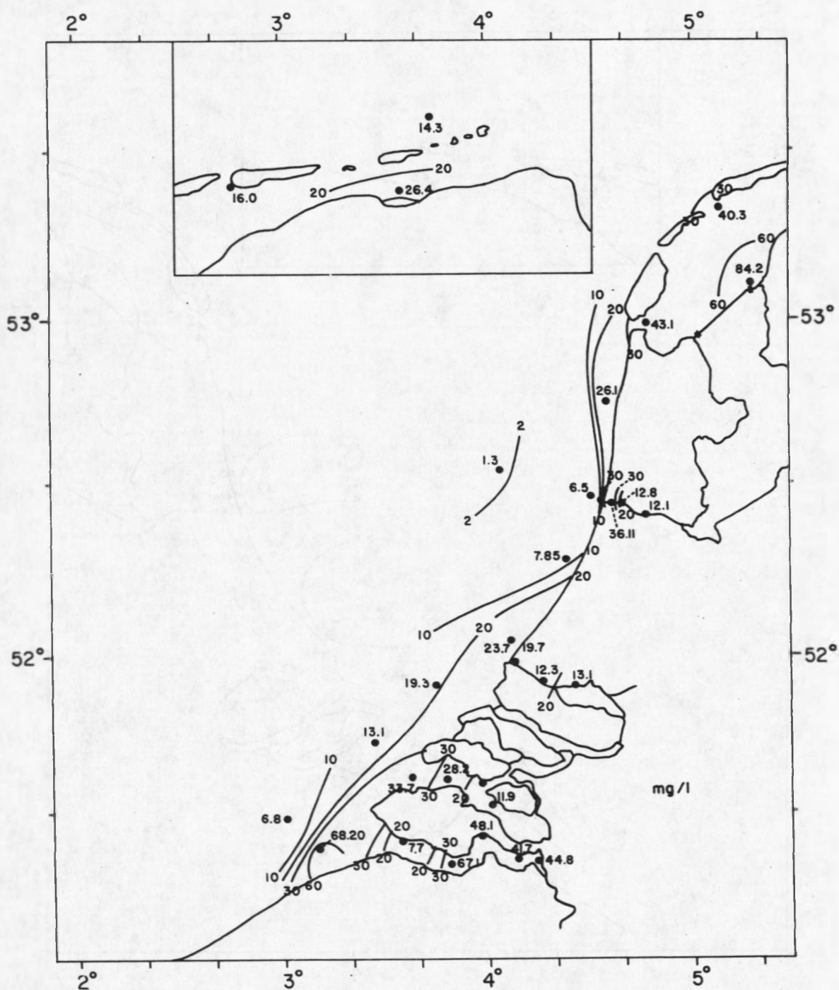
Fig. 11. Gesuspendeerd materiaal ( \text{mg.l}^{-1} ), januari 1986.
