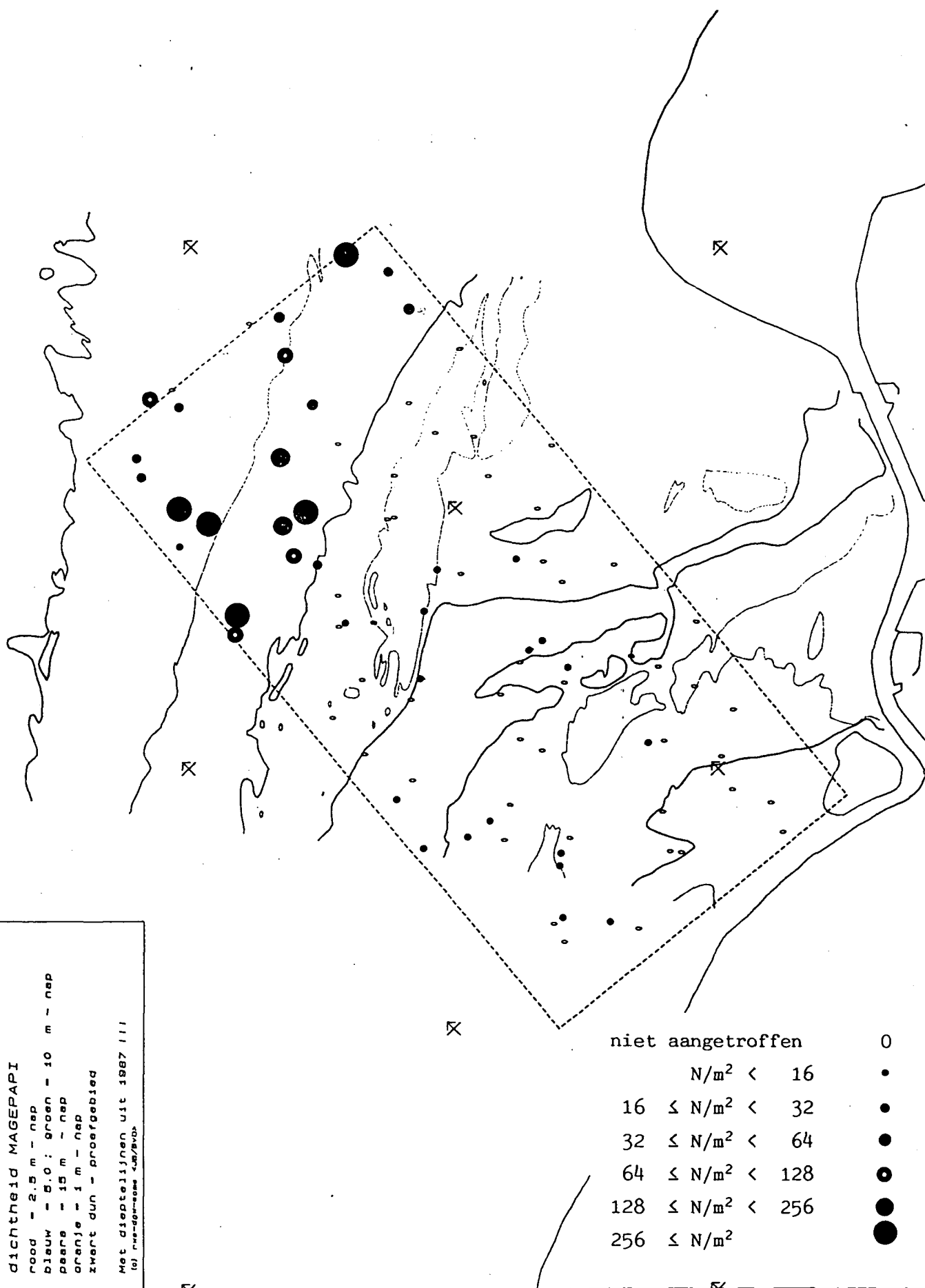
Figuur 29.b Dichtheid Magelona papillicornis (Grevelingengebied)
