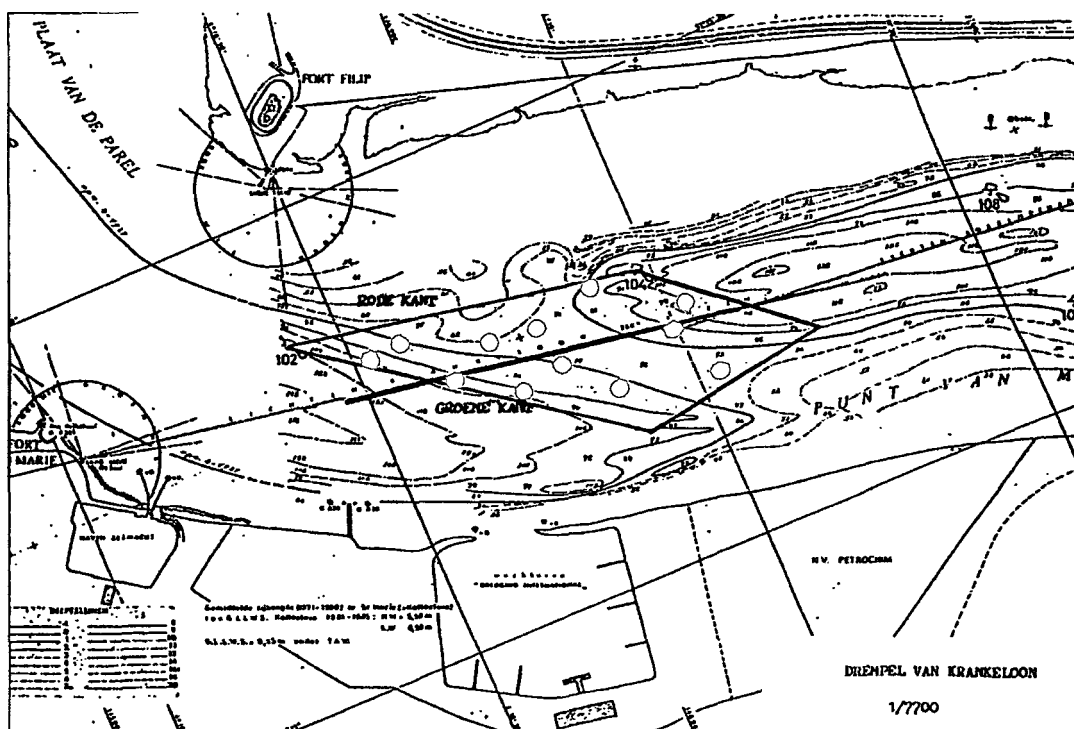
Figuur 1: Voorbeeld van staalname op de drempel van Krankeloon. Aan iedere kant van het vaarwater werd een mengstaal genomen, telkens bestaande uit 6 grepen met een Van Veengripper
