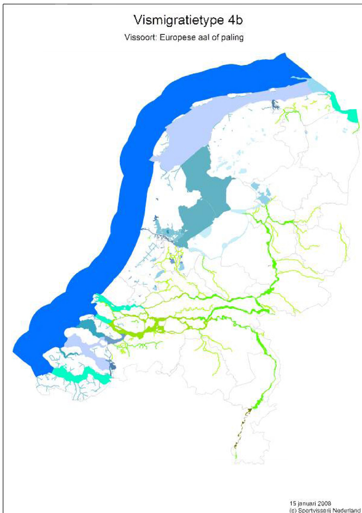
figuur 2.10 Resultaat van de selectie van K, O, grote R en vlakvormige M-typen voor het migratietype 4B.
