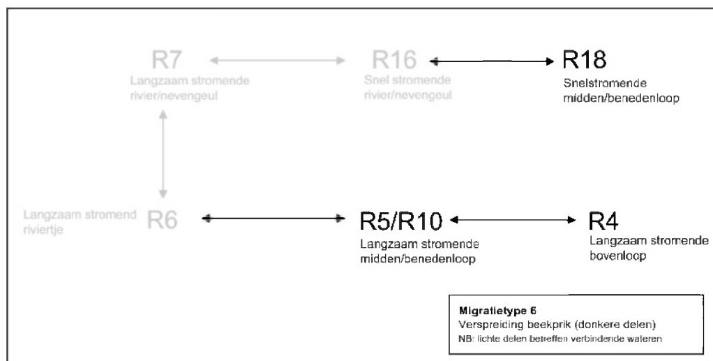
figuur 2.14 Schematische voorstelling van het verspreiding van beekprik binnen KRW-typen. In grijsstinten zijn de mogelijke verbindingen weergegeven tussen de relevante R-typen.
