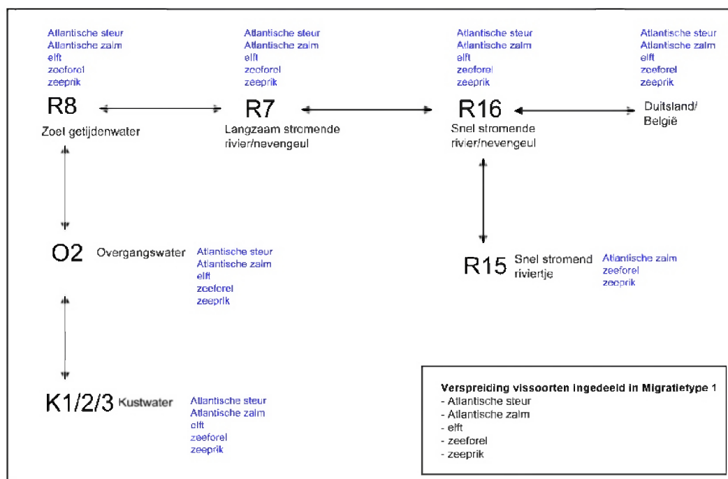
figuur 2.1 Schematische voorstelling van het verspreiding van Atlantische steur, Atlantische zalm, elft, zeeforel en zeeprink binnen KRW-typen.
