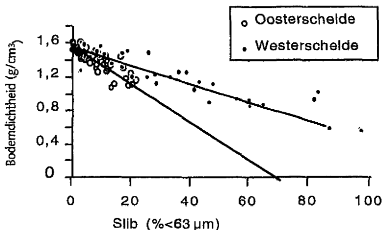
Figuur 2. Relatie slibgehalte (% sedimentdeeltjes < 63 µm) en bodemdichtheid (soortelijk gewicht van de bodem). De relatie voor de Westerschelde wordt beschreven door de vergelijking y = -0.01x + 1.54 ( R^2 = 0.85 ) en die voor de Oosterschelde door de vergelijking y = -0.02x + 1.57 ( R^2 = 0.51 ), waarin y = bodemdichtheid en x = slibgehalte.
