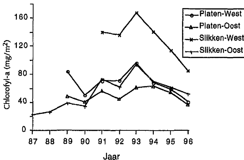
Figuur 7. Verloop van het jaargemiddeld chlorofyl-a gehalte ( \text{mg m}^{-2} ) van alle monsterpunten in de Westerschelde vanaf 1988 t/m 1996, ingedeeld in 4 gebieden: Slikken West, Platen West, Slikken Oost en Platen Oost.
