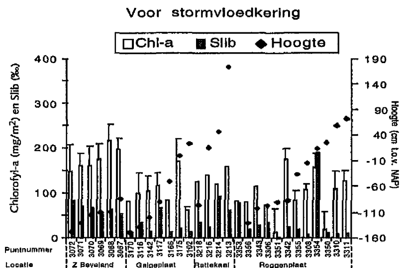
Figuur 3a. Gemiddeld chlorofyl-a gehalte ( \text{mg m}^{-2} ; witte staafjes + 1 sd), gemiddeld slibgehalte (% (l) fractie < 63 \mu\text{m} ; grijze staafjes) en de gemiddelde hoogteligging (cm t.o.v. NAP; zwarte punten) voor de verschillende monsterpunten in de Oosterschelde voor (A) en na (B) de bouw van de stormvloedkering. In tabel 2 is voor de verschillende monsterpunten aangegeven of het punt in 1989 een hoog- (H) of een laagdynamisch (L) karakter heeft.
