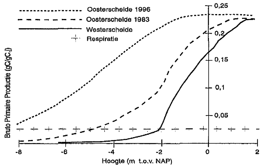
Figuur 9a Bruto primaire productie microfytobenthos in relatie tot plot hoogte (mm t.o.v. NAP). A: gemiddelde bruto jaarproductie in \text{gC}^{-1} \text{ j}^{-1} . De stippe lijn representeert het niveau van de respiratie van microfytobenthos. B: gemiddelde jaarproductie in \text{gC m}^{-2} \text{ j}^{-1} . Voor de relatie tussen A en B zie Intermezzo I.
