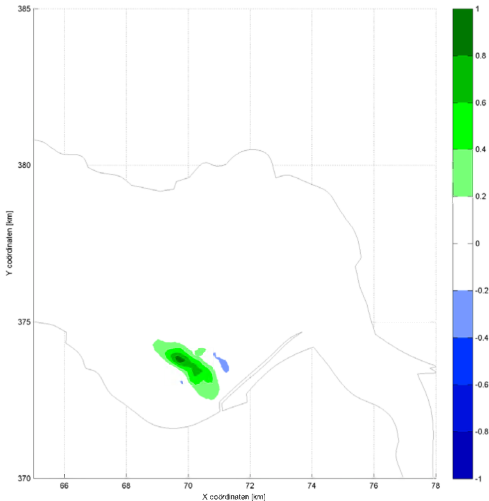
Figuur 7.4 Verschil in maximale stroomsnelheid tijdens vloed
