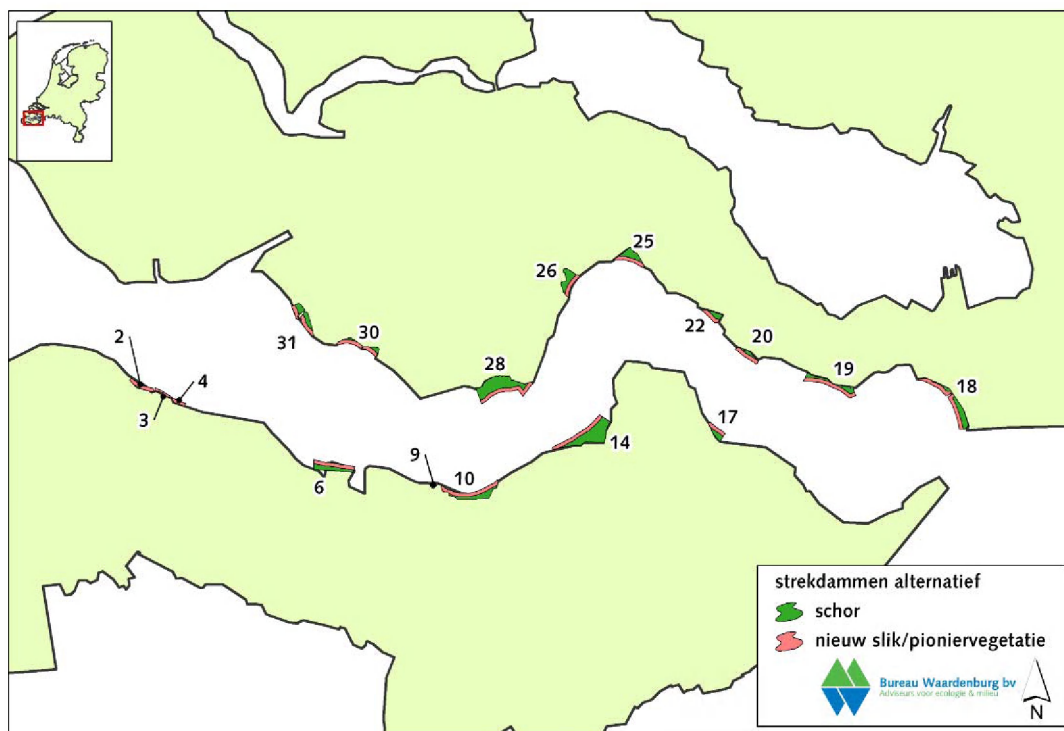
Figuur 6.1 Overzicht morfologisch kansrijke locaties uitvoeringsvariant buitendijkse schorontwikkeling (exclusief locaties project Middengebiet)
