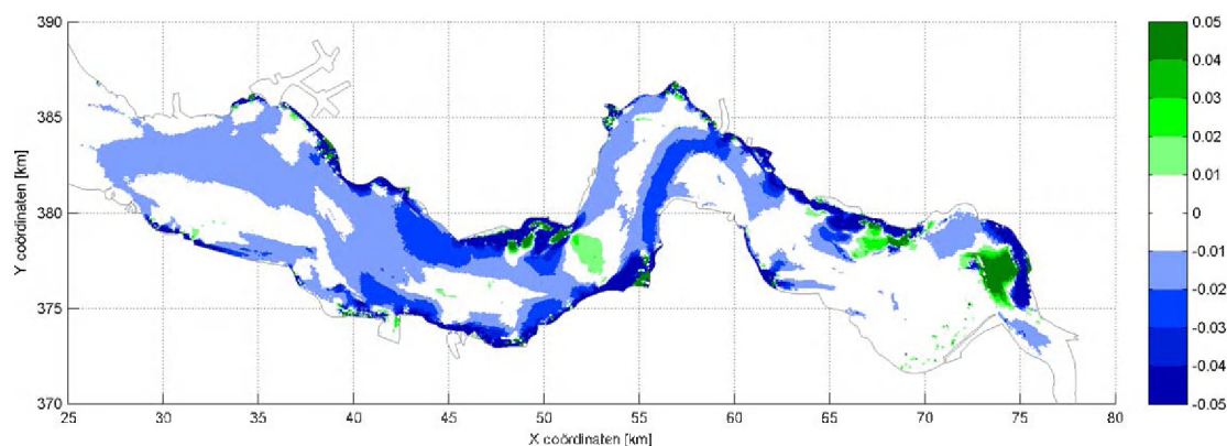
Figuur 6.6 Verschil in maximale stroomsnelheden bij eb in m/sec
