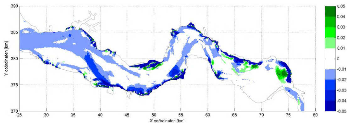
Figuur 6.5 Verschil in maximale stroomsnelheden bij vloed in m/sec
