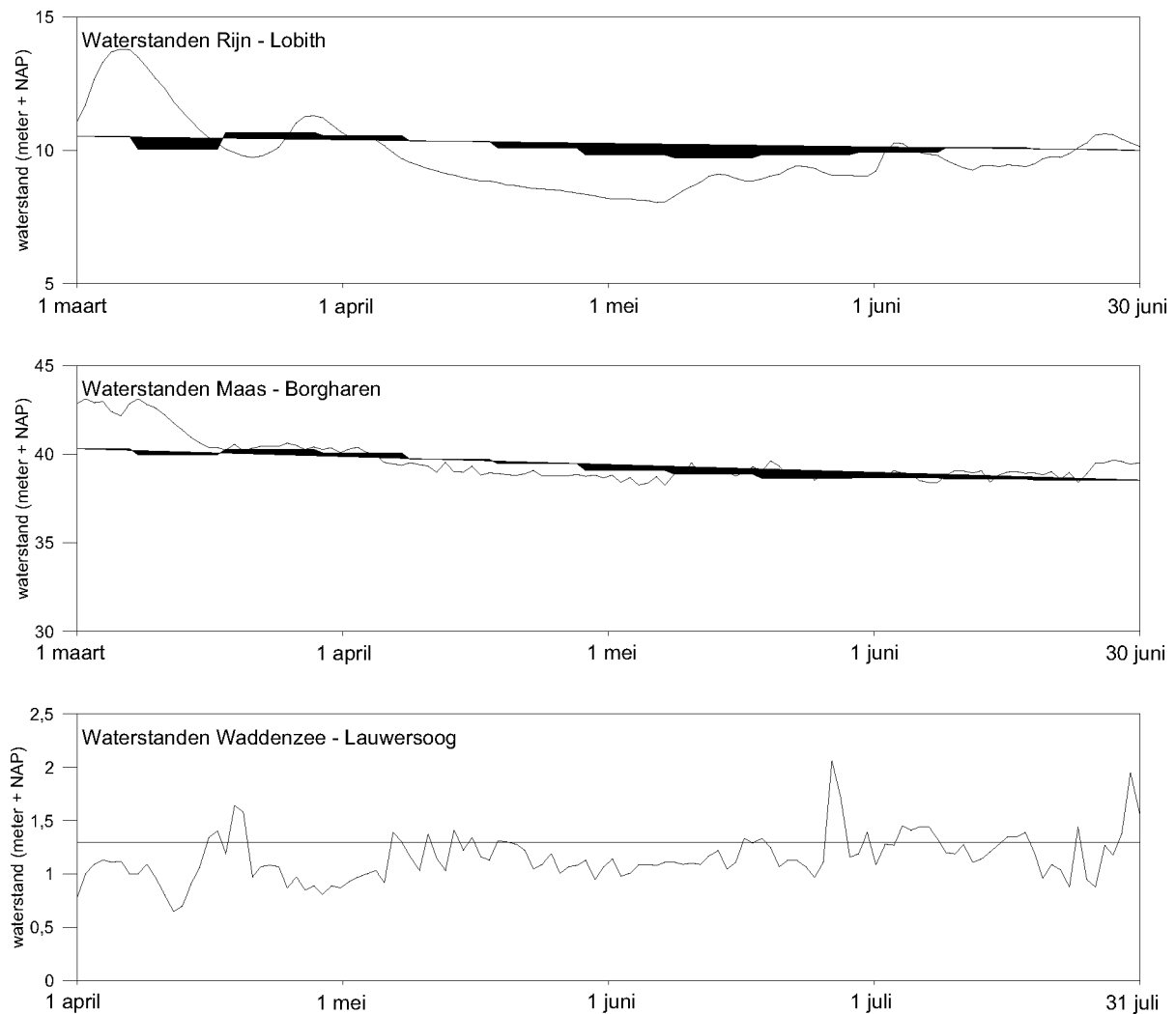
Figuur 3.2. Waterstanden in Rijn (Lobith) en Maas (Borgharen) in maart-juni 2007 en waterstanden in de Waddenzee (Lauwersoog) in april-juli 2007 (Rijkswaterstaat, www.waterbase.nl ). Voor de rivieren zijn actuele metingen (dikke lijn) vergeleken met het lange termijn gemiddelde (stippellijn); voor de Waddenzee is het hoogste tij per dag aangegeven. De stippellijn geeft aan bij welk tij de meeste landaanwinningsswerken overspoelen. / Water tables in Rivers Rhine (Lobith) and Meuse (Borgharen) and in the Wadden Sea. For the rivers, daily values (solid line) are compared with long-term averages (dashed line). For the Wadden Sea the dashed line marks the tide that leads to inundation of (lower) salt marshes.
