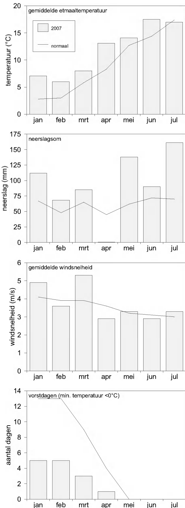
Figuur 3.1. Samenvatting van het weer gedurende het eerste halfjaar van 2007, afgeleid uit gegevens van het KNMI-station De Bilt ( www.knmi.nl ). Weergegeven zijn de actuele weersmetingen en de lange termijn waarden ('normalen') in 1971-2000. / Weather characteristics during the breeding season 2007. Shown are mean daily temperatures, precipitation, average windspeed and the number of days with temperatures below zero. Bars indicate actual values in 2007, lines long term averages.
