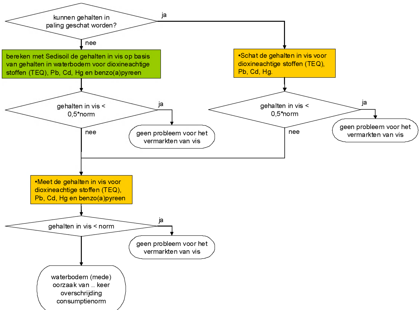
Figuur 4.9 Schema voor toetsing aan consumptienormen.
