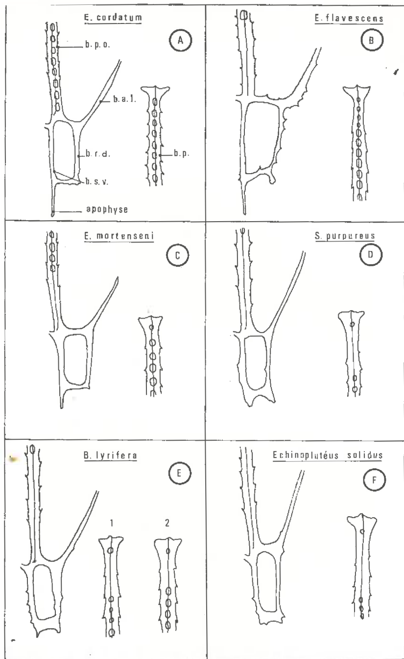
FIG. 5. — Squelette des échinoplutés d' Echinocardium cordatum , Echinocardium flavescens , Echinocardium mortenseni , Spatangus purpureus , Brissopsis lyrifera et de l' echinopluteus solidus au stade IV bras. Vue latérale.
