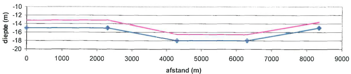
ebgeul, 5% storten + comp. Baggeren, Symm. Cel, niet-uniforme geulgeometrie.
