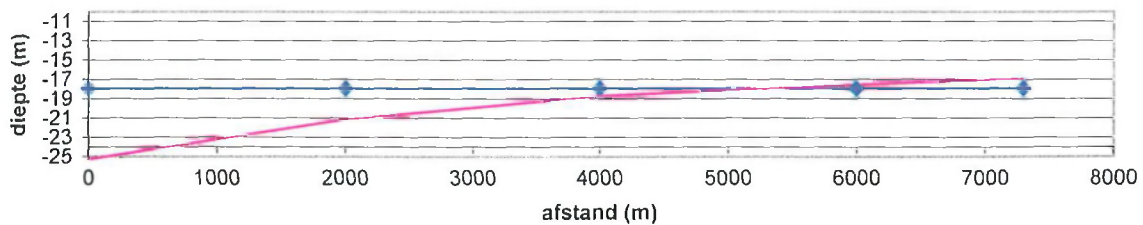
ebgeul, 5% storten in ebgeul + comp. baggeren buiten cel; Symm. Cel, niet-uniforme geulgeometrie.
