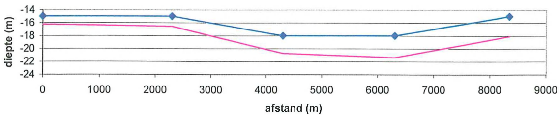
Vloedgeul, 5% storten + comp. Baggeren, Symm. Cel, niet-uniforme geulgeometrie.
