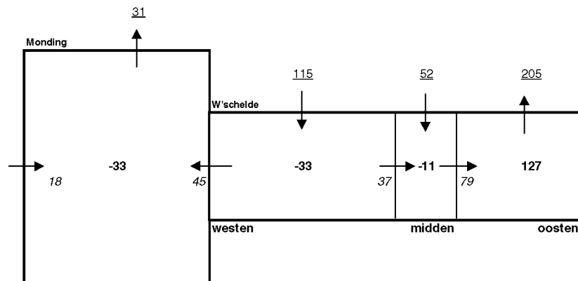
Fig. 3.4 Zand/waterbalans t.o.v. NAP+2m over de totale periode 1999-2030 na derde verdieping , variant a. V_{\text{tot,E}} = vet, totale inhoudsverandering berekend door ESTMORF, V_i = onderstreept, totale netto ingreep. I/E = cursief, import/ export van zanduit tussen deelgebieden.
