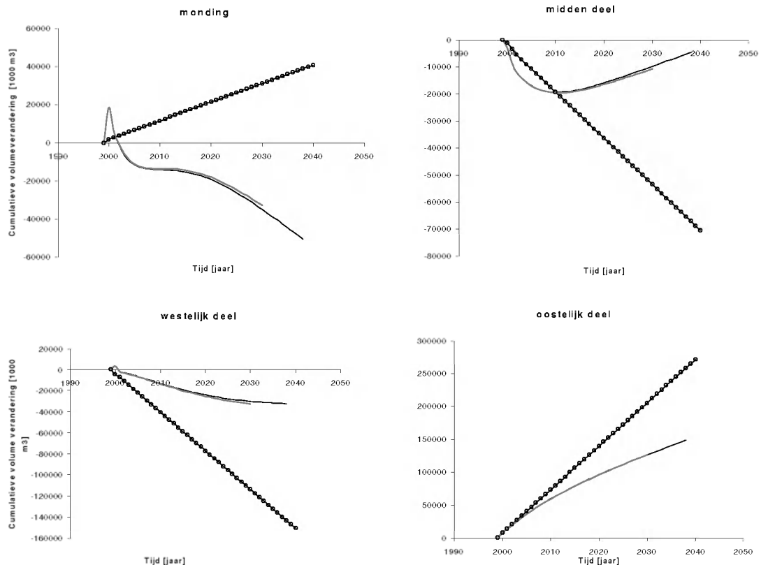
Figuur 3.9 Tijdreeksen van de cumulatieve totale inhoudsveranderingen V_{tot} (—) en de netto ingrepen V_i (-o-) als gevolg van de zeespiegelstijging. Grijs lijn is V_{tot} zonder zeespiegelstijging (Fig.3.1).
