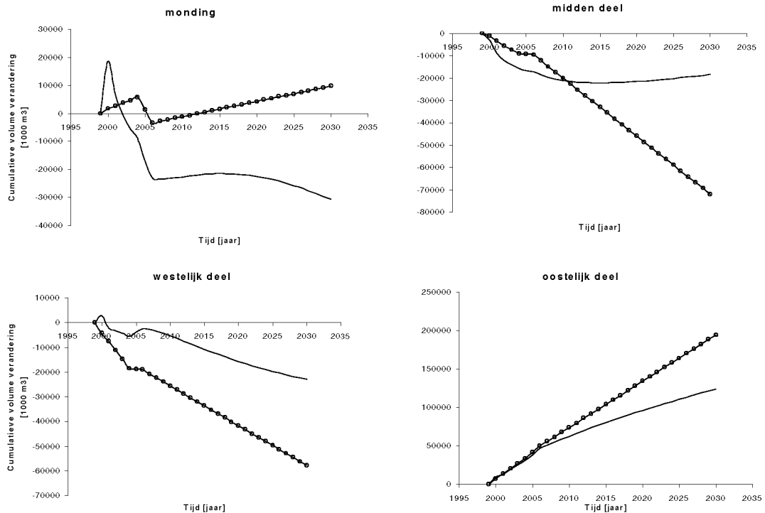
Figuur 3.7 Tijdreeksen van de cumulatieve totale inhoudsveranderingen V_{\text{tot}} (—) en de netto ingrepen V_i (-o-) als gevolg van de derde verdieping , variant c.
