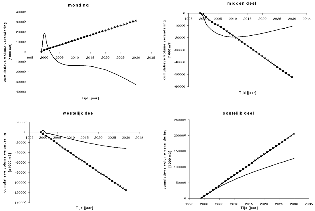
Figuur 3.3 Tijdreeksen van de cumulatieve totale inhoudsveranderingen V_{\text{tot}} (—) en de netto ingrepen V_i (-o-) als gevolg van de derde verdieping , variant a.
