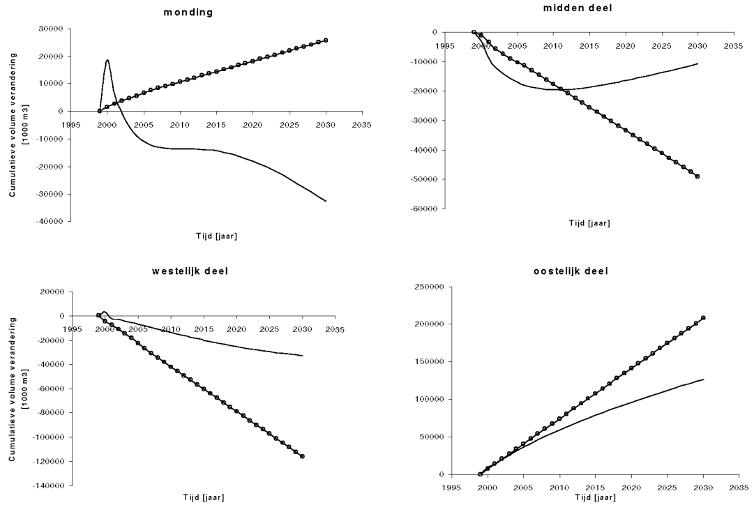
Figuur 3.5 Tijdreeksen van de cumulatieve totale inhoudsveranderingen V_{tot} (—) en de netto ingrepen V_i (-o-) als gevolg van de derde verdieping, variant b .
