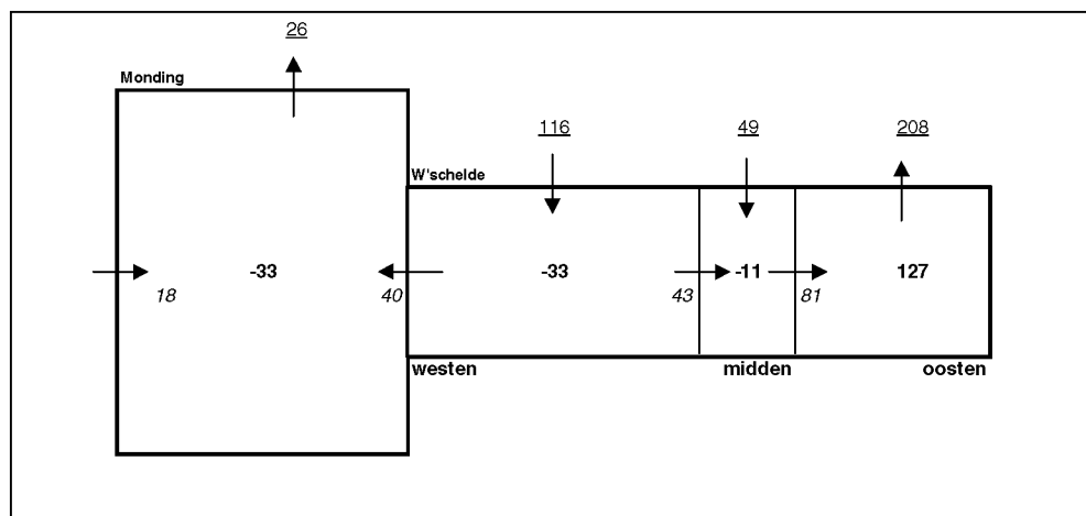
Fig. 3.6 Zand/waterbalans t.o.v. NAP+2m over de totale periode 1999-2030 na derde verdieping, variant b . V_{tot,E} = vet, totale inhoudsverandering berekend door ESTMORF, V_i = onderstreept, totale netto ingreep. I/E = cursief, import/ export van zanduit tussen deelgebieden.
