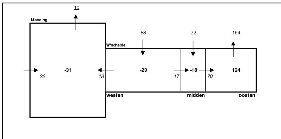
Fig. 3.8 Zand/waterbalans t.o.v. NAP+2m over de totale periode 1999-2030 na derde verdieping , variant c. V_{\text{tot,E}} = vet, totale inhoudsverandering berekend door ESTMORF, V_i = onderstreept, totale netto ingreep. I/E = cursief, import/ export van zanduit tussen deelgebieden.
