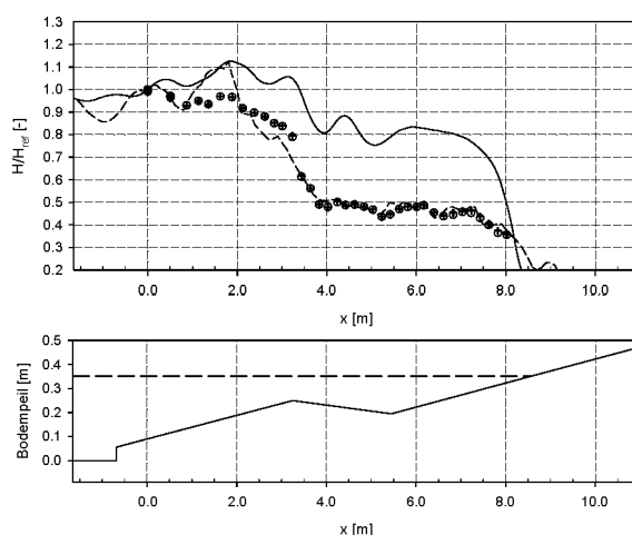
Figuur 2. Run 13 (drempel-dal profiel, schaal 0.5); (a) experimentele resultaten ('o' en '+' tekens), MILDwave resultaten (volle lijn), SimWave resultaten (stippellijn); (b) bodemprofiel.
