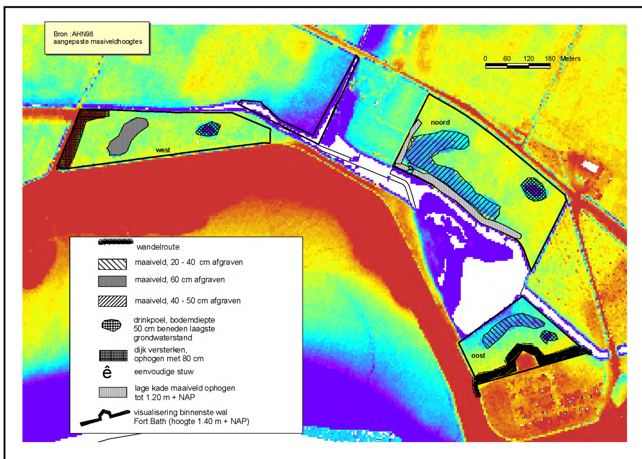
Figuur 12: Inrichtingsmaatregelen
