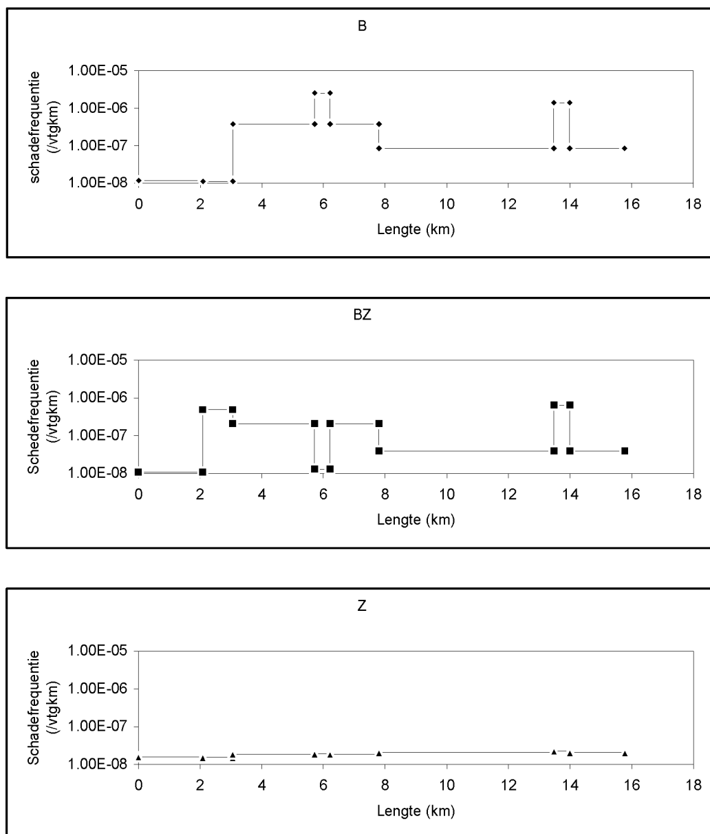
Figuur 3. Verloop scheepsschadefrequentie langs het Kanaal van Gent naar Terneuzen (0=Westerschelde, 16=grens België; B=binnenvaart; BZ=Binnenvaart-Zeevaart; Z=Zeevaart)
