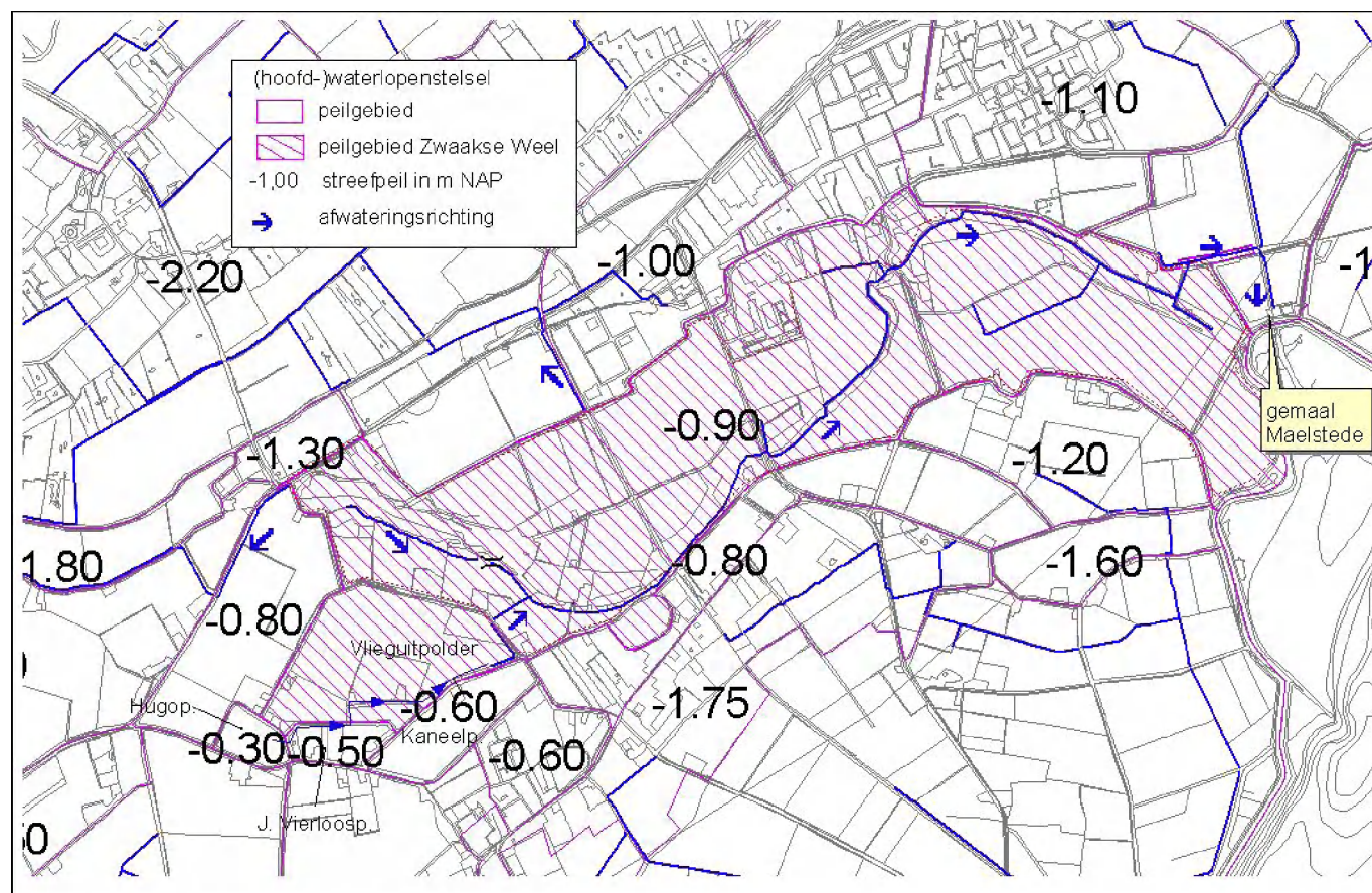
Figuur 9. (Hoofd-)afwateringssysteem
