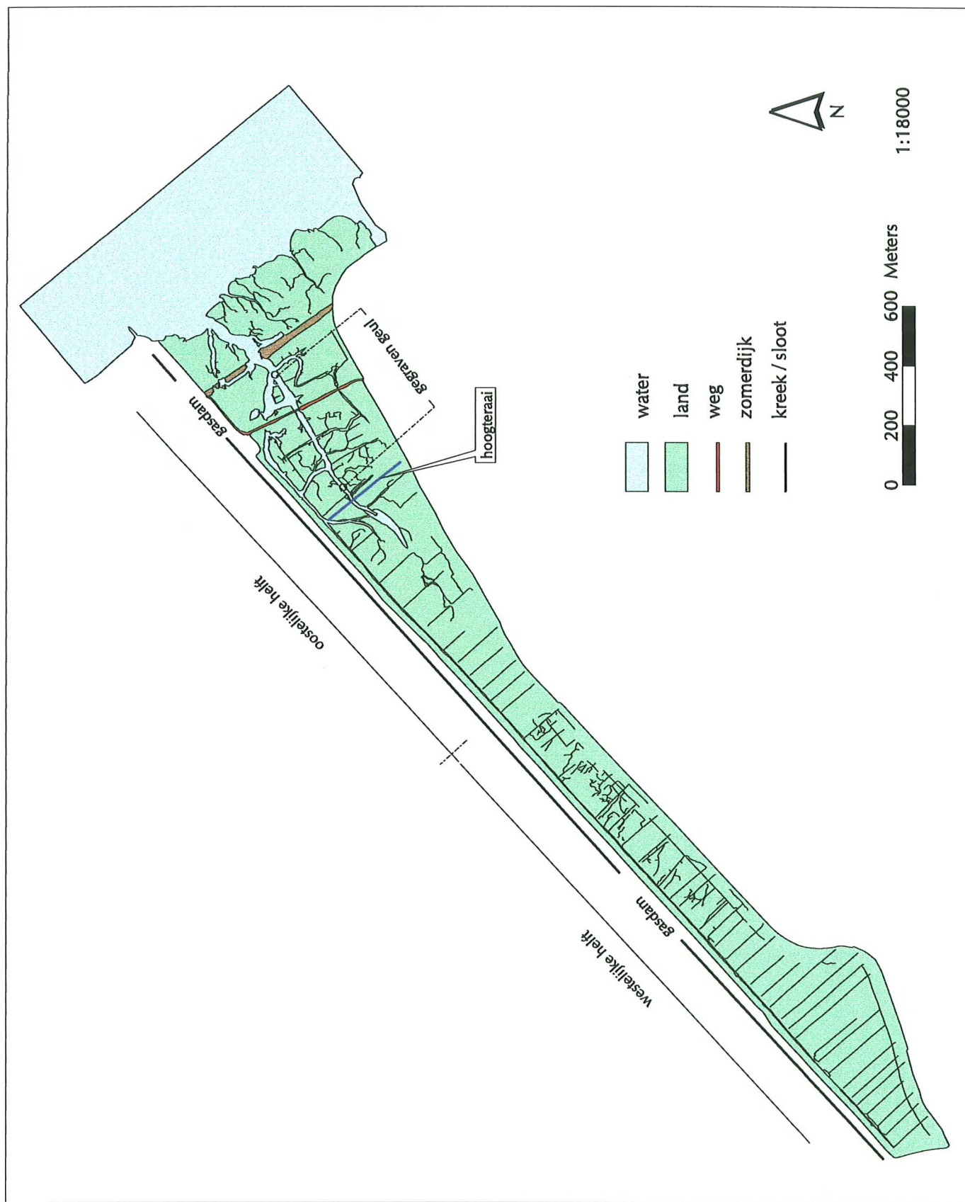
Fig. 2.3 Kreen- en afwateringspatroon Sieperdaschor 1995
