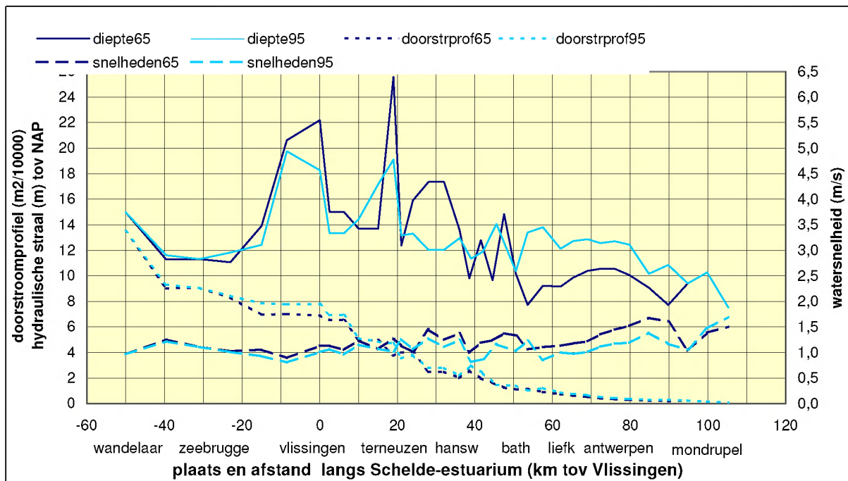
fig. 6.7 veranderingen 1965-1995 diepte / hydraulische straal, doorstroombroef en met HARMSCHEDES gesimuleerde snelheden
