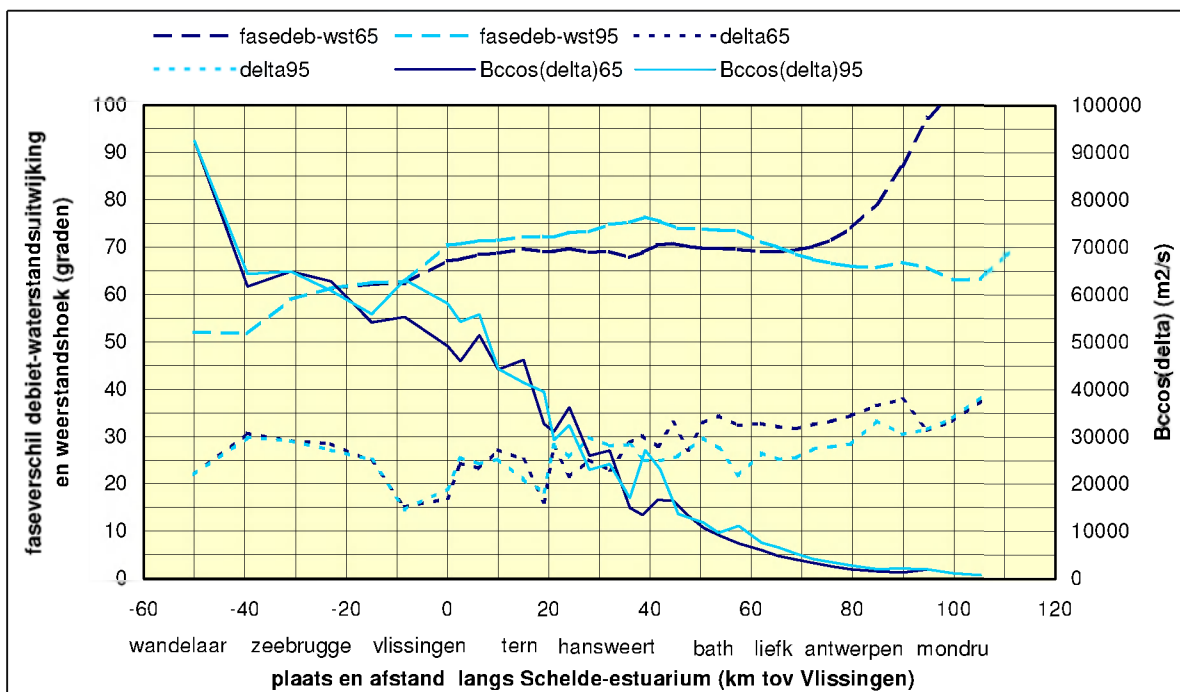
fig 6.9 veranderingen 1965-1995 faseverschil tussen debiet en waterstandsuitwijking, reflectie- factor en weerstandshoek, gesimuleerd met HARMSCHDELDE96/95
