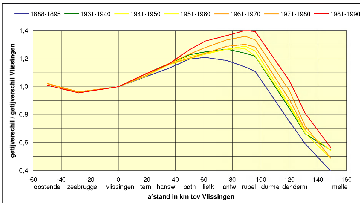
fig. 5.12 de versterking van het getijverschil bij gemiddeld getij ten opzichte van Vlissingen; ontwikkeling over 1941-1990 vergeleken met 1888-1940
