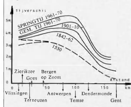
Figuur 10: Tijverschillenverloop Schelde in langszin.
