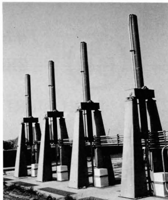
Hydraulische aandrijving van de 4 schuiven van de langsrivol.
