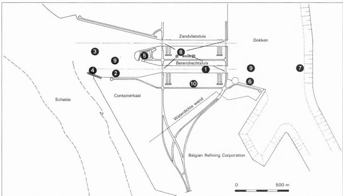
Fig. 2: 1 sluis, 2 zuidelijke kaaimuur, 3 afgebroken kaaimuur, 4 pier (caisson-methode), 5 schuilhaven, 6 wachtkade, 7 bochtverbreding tussen Kanaaldok B2 en B3, 8 basculebruggen, 9 baggerwerken van de toegangseculen, 10 bijhorende wegenwerken.
