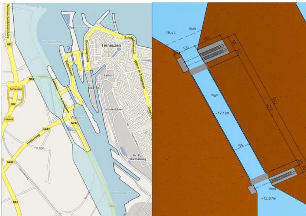
Figuur 12-1 Nieuwe zeesluis buiten complex (ten westen van huidige grote zeesluis)
