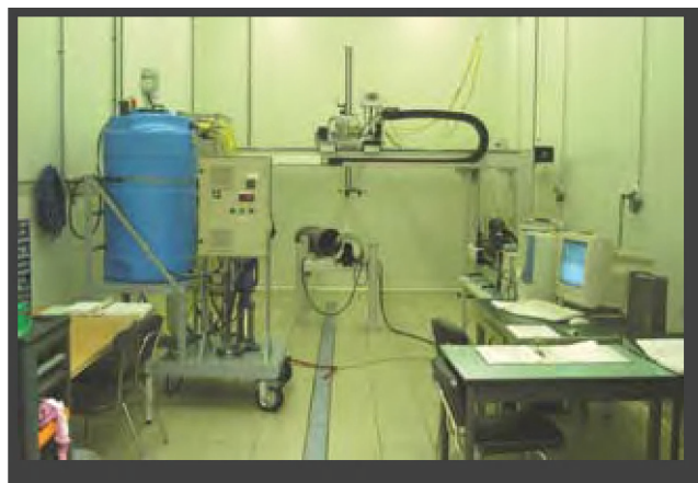
PDPA-laser meetopstelling voor het opmeten van druppelsnelheden en -groottes van spuitdoppen
