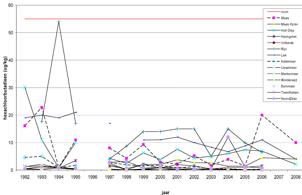
Figuur 9. Concentraties van hexachloorbutadieen in aal in verschillende Nederlandse wateren.
