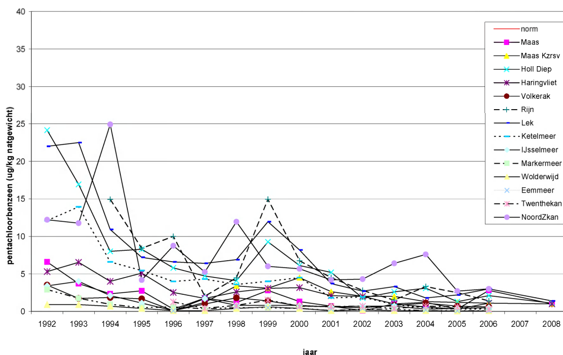
Figuur 12. Concentraties van pentachloorbenzeen in aal in verschillende Rijkswateren. De norm ( MKN_{biota} ) voor pentachloorbenzeen is niet in de figuur weergegeven en betreft 367 \mu\text{g/kg} .
