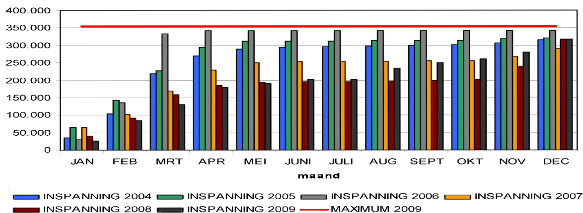
Grafiek 23: Cumulatieve visserij-inspanning in ICES-gebied VII-Schelpen
