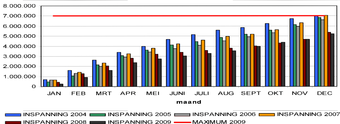
Grafiek 22: Cumulatieve visserij-inspanning in ICES-gebied VII
