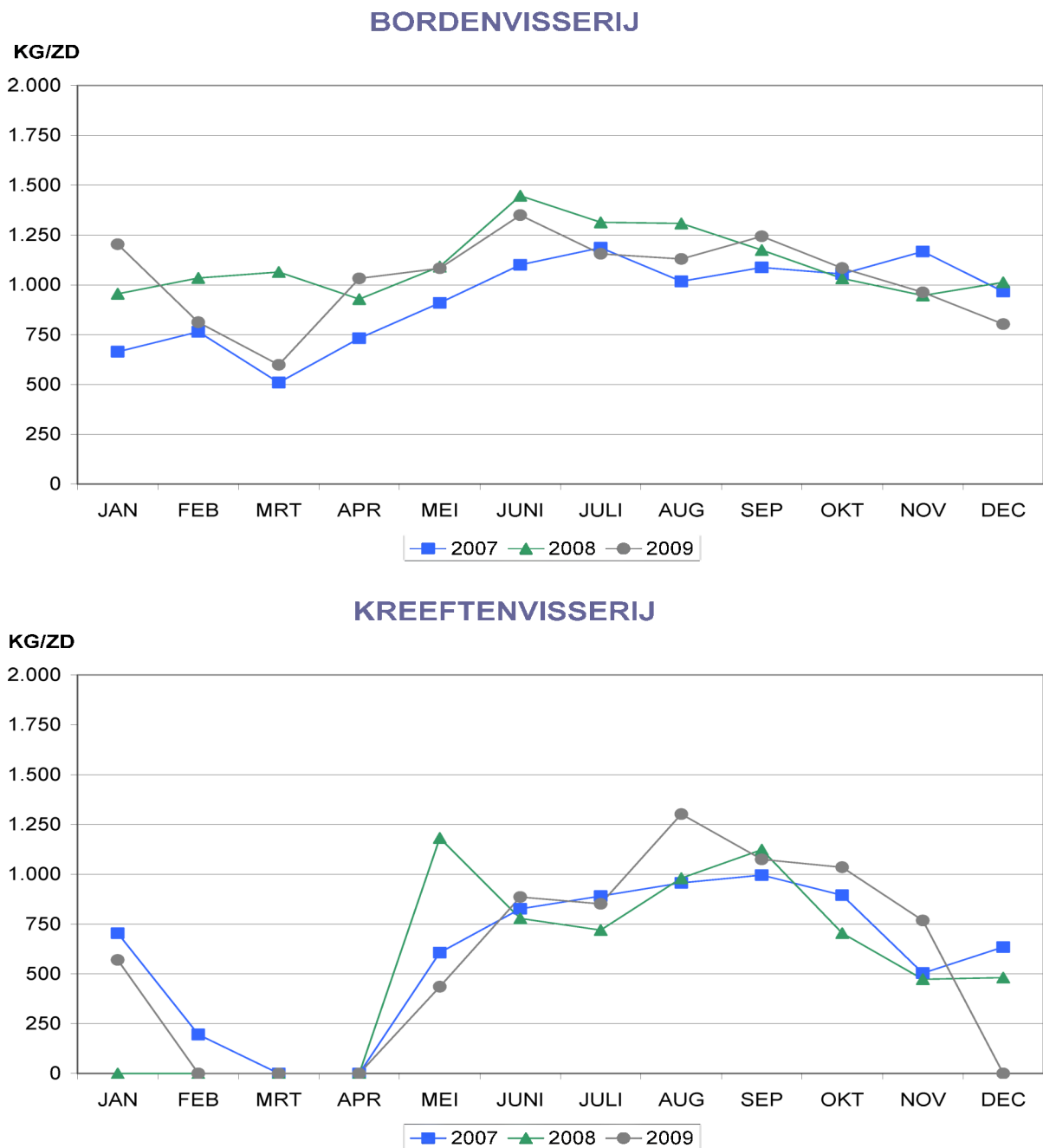
Grafiek 19: Maandelijks aanvoer per zeedag per visserij in Belgische + vreemde havens
