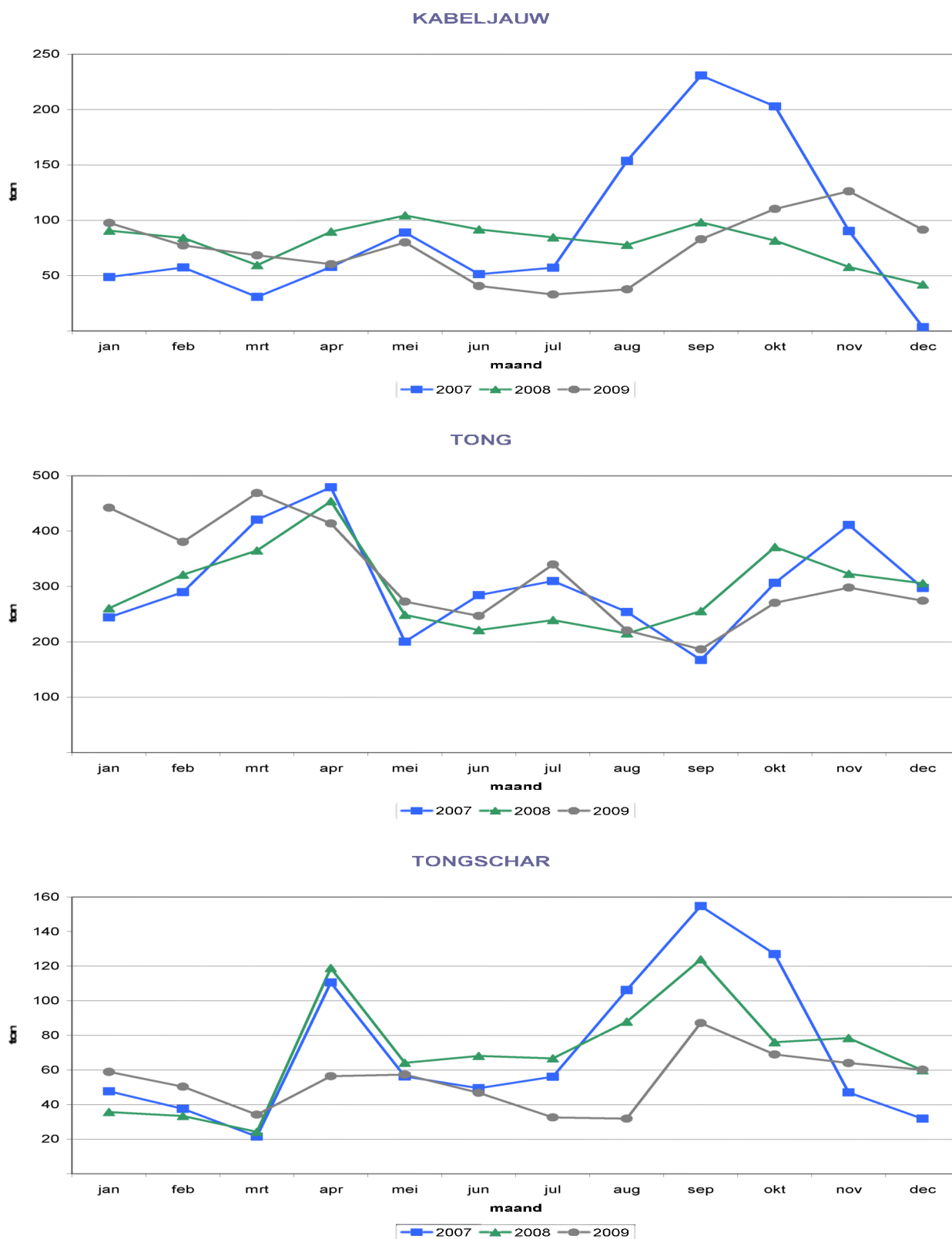
Grafiek 7 : Maandelijks aanvoer per vissoort in Belgische + vreemde havens
