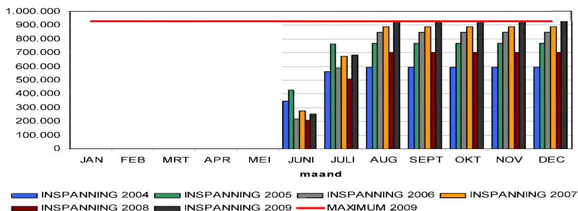
Grafiek 24: Cumulatieve visserij-inspanning in ICES-gebied VIII
