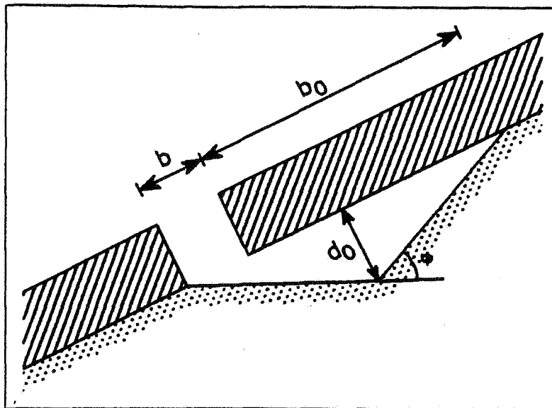
Schematisatie erosiekuil
