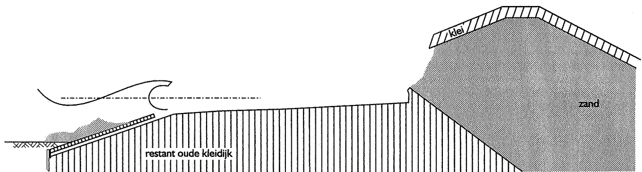
5a. Zandkern deels onbeschermd maar niet aan directe golfaanval blootgesteld
