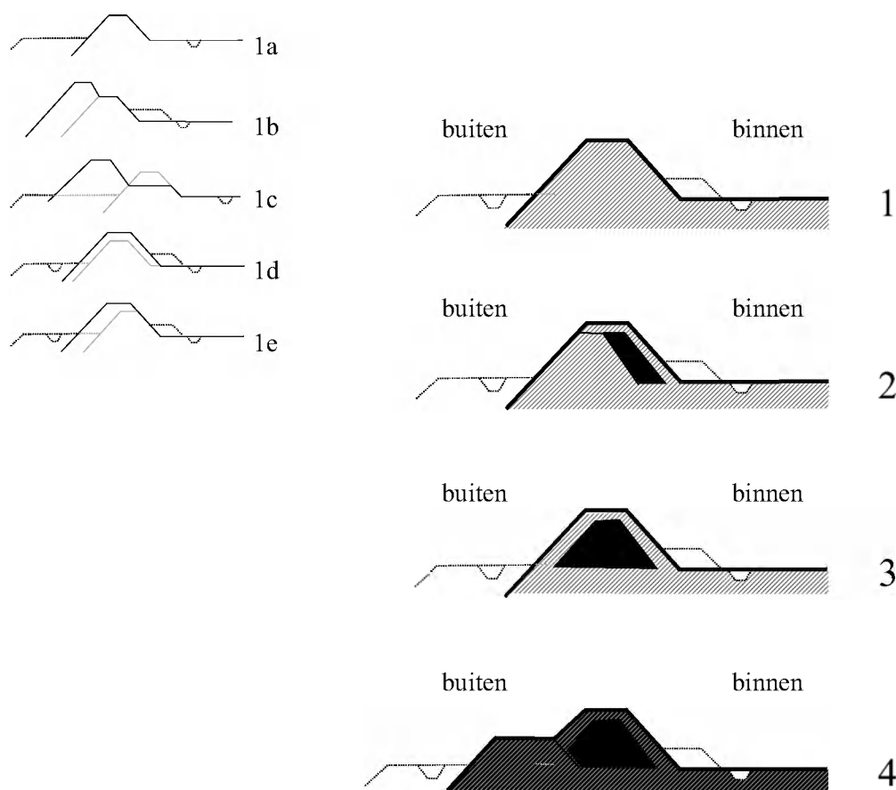
Figuur 2.5: Geschematiseerde karakteristieke dwarsprofielen van dijken in Nederland
