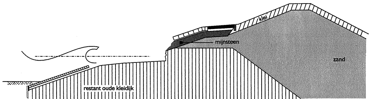
4a. Kleikern wordt aan directe golfaanval blootgesteld, erosie kleikern
