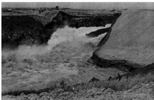
Teton Dam Faaltraject van primaire microinstabiliteit tot een doorbraak in het plaatje rechtsonder
