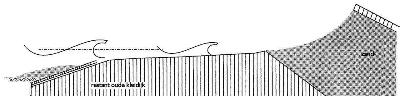
6a. Kleikern geerodeerd, zandkern aan directe golfaanval blootgesteld
