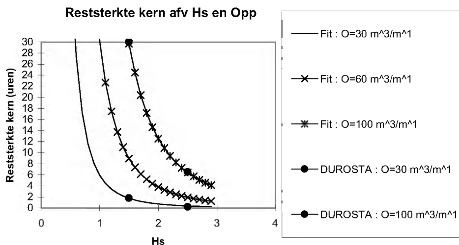
Figuur 8.18 Reststerkte van het kernmateriaal als functie van het te eroderen oppervlak boven de waterlijn
