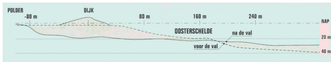
Figuur 9.2 Dijkval
