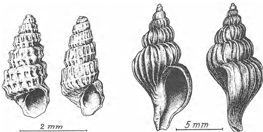
Ividella excavata
