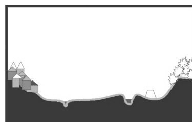
Fig. 1: De opbouw van de Dijlevallei te Neerijse
